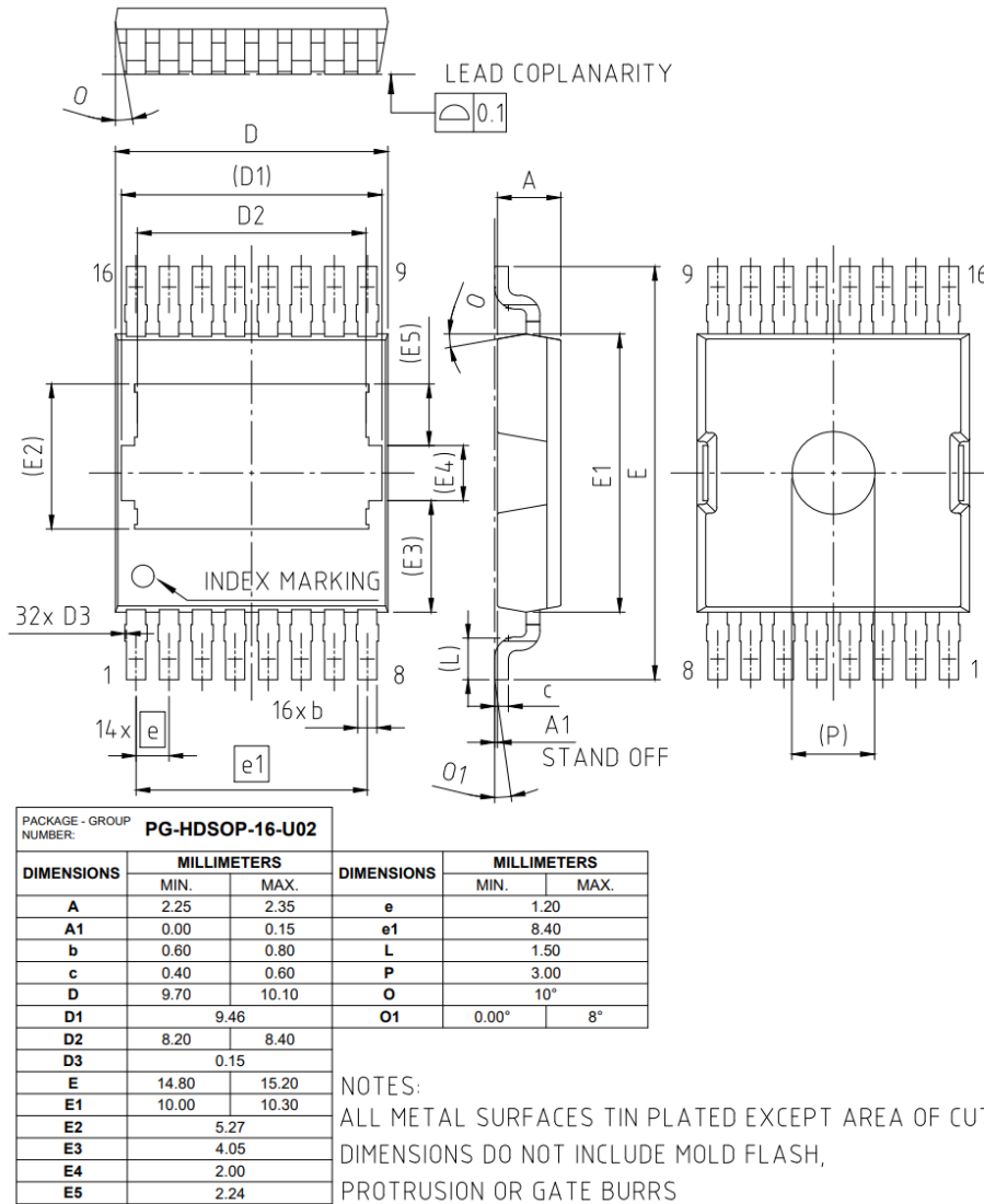
图 1 PG-HDSOP-16 外形图，尺寸单位为毫米
