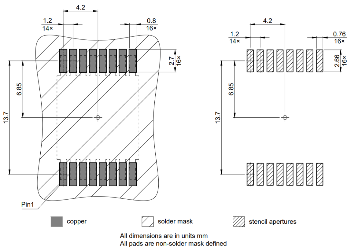
图 2 PG-HDSOP-16 封装图，尺寸单位为毫米
