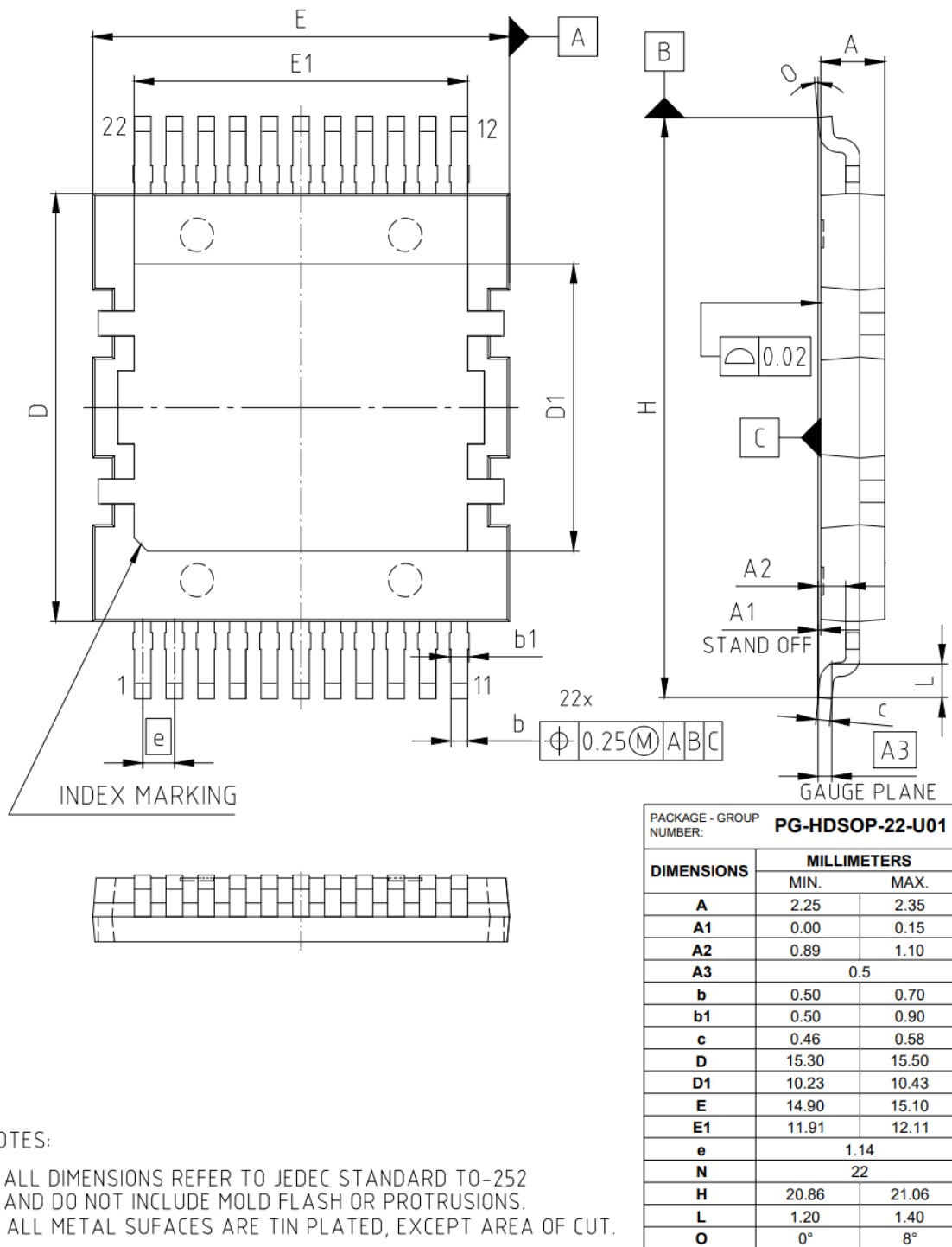
图 1 PG-HDSOP-22 外形图，尺寸单位为毫米
