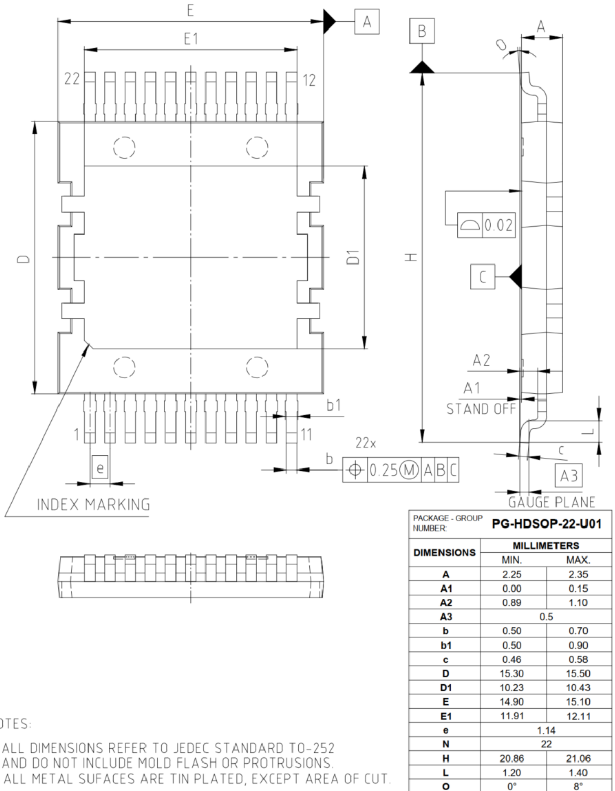
图 1 PG-HDSOP-22 外形图，尺寸单位为毫米
