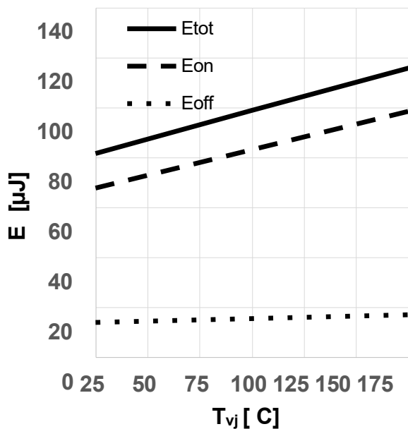
图 15 典型开关能量损耗随结温变化关系
