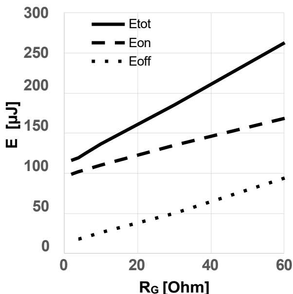
图 17 典型开关能量损耗随栅极电阻变化关系 (E = f(R_{G,ext}), V_{DD} = 800V, V_{GS} = 0V/18V, I_D = 6A, T_{vj} = 175^\circ C, \text{独立负载, 测试电路见图 E, 二极管: } V_{GS} = 0V \text{ 时的体二极管})
