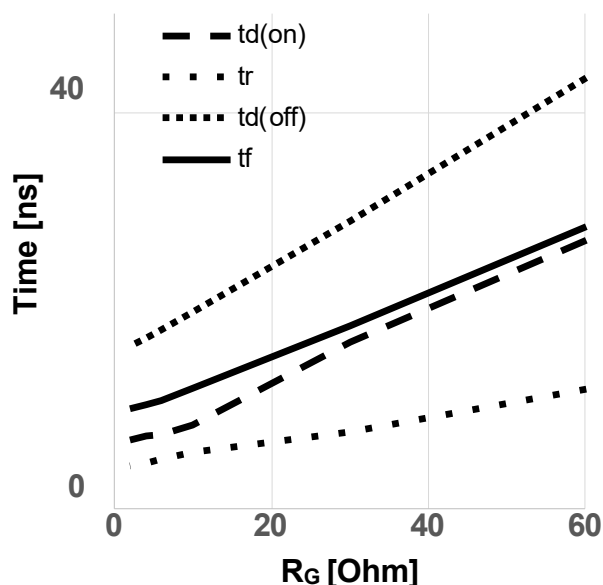
图 18 典型开关时间随栅极电阻变化关系 (t = f(R_{G,ext}), V_{DD} = 800V, V_{GS} = 0V/18V, I_D = 6A, T_{vj} = 175^\circ C, \text{独立负载, 测试电路见图 E, 二极管: } V_{GS} = 0V \text{ 时的体二极管})
