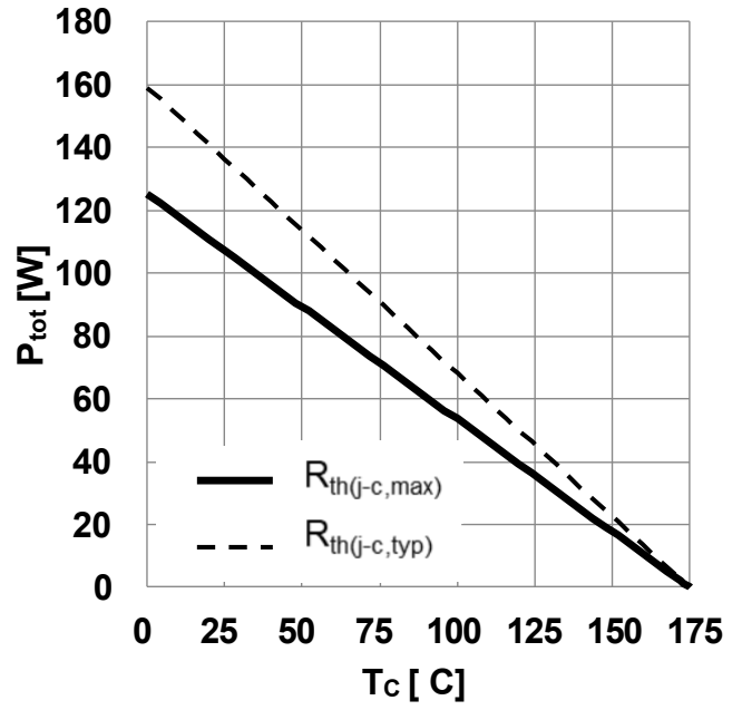
图 2 功率耗散随壳温 (受限于接合线) 变化关系 ( P_{tot} = f(T_c) )
