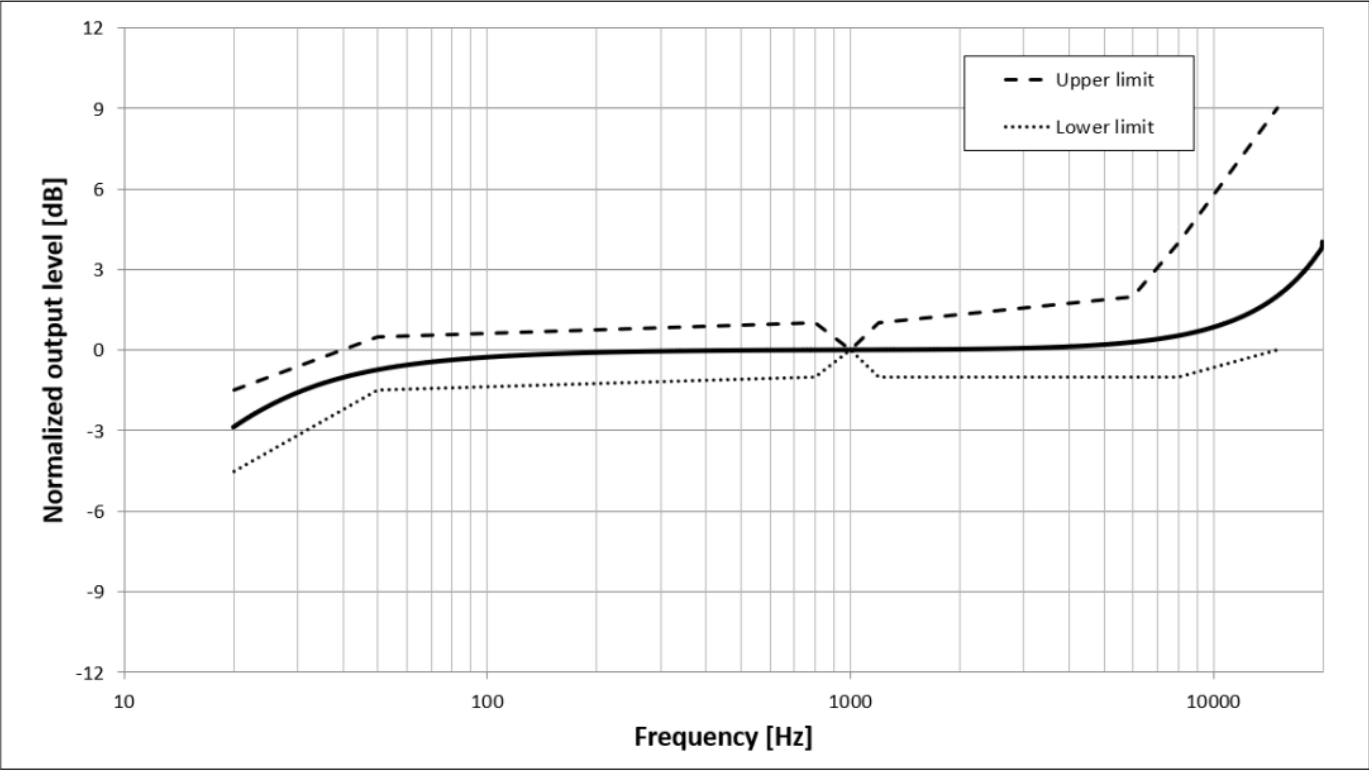
图10 IM73A135V01自由场频率响应
