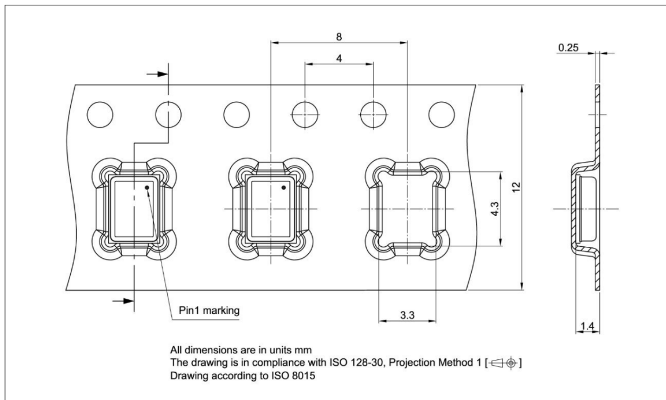
图14 IM73A135V01卷带包装信息
