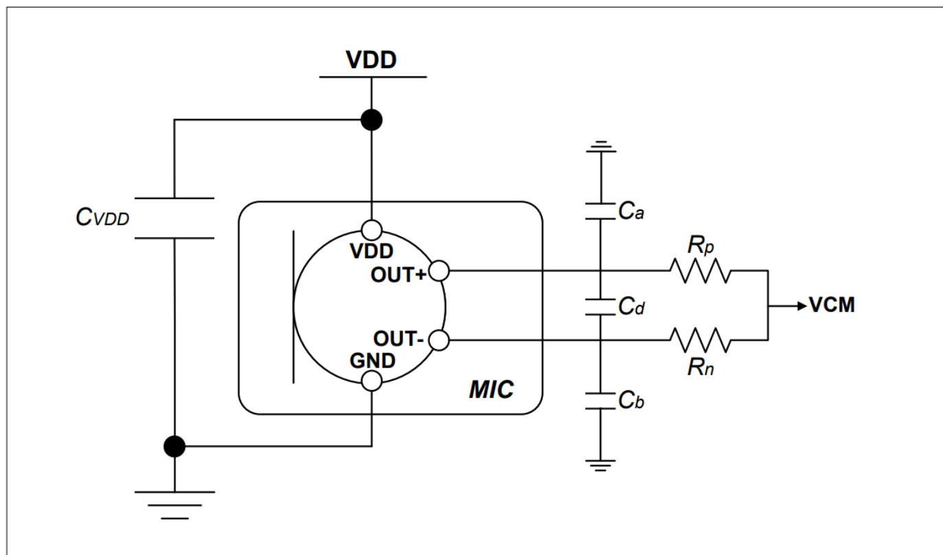
图11 输出负载配置
