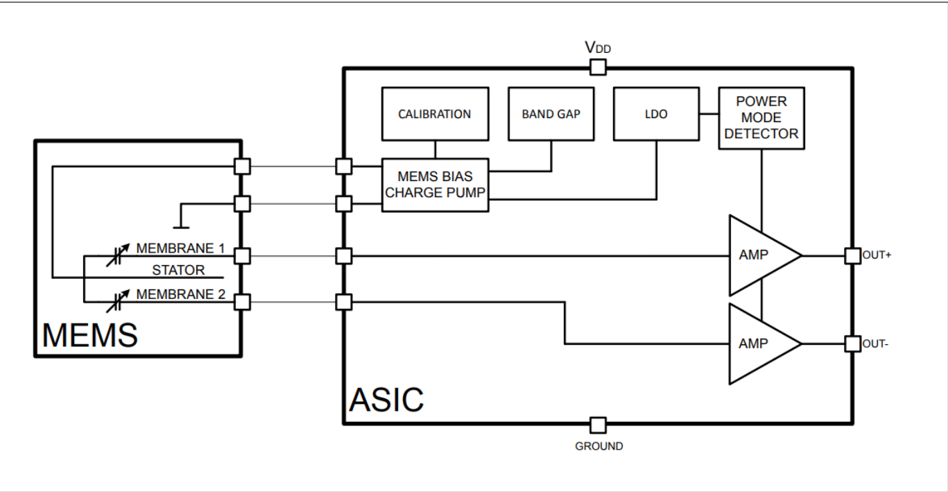
图1 IM73A135V01框图
