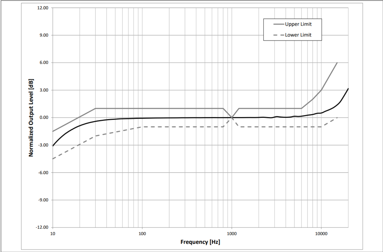
图10 自由场频率响应
