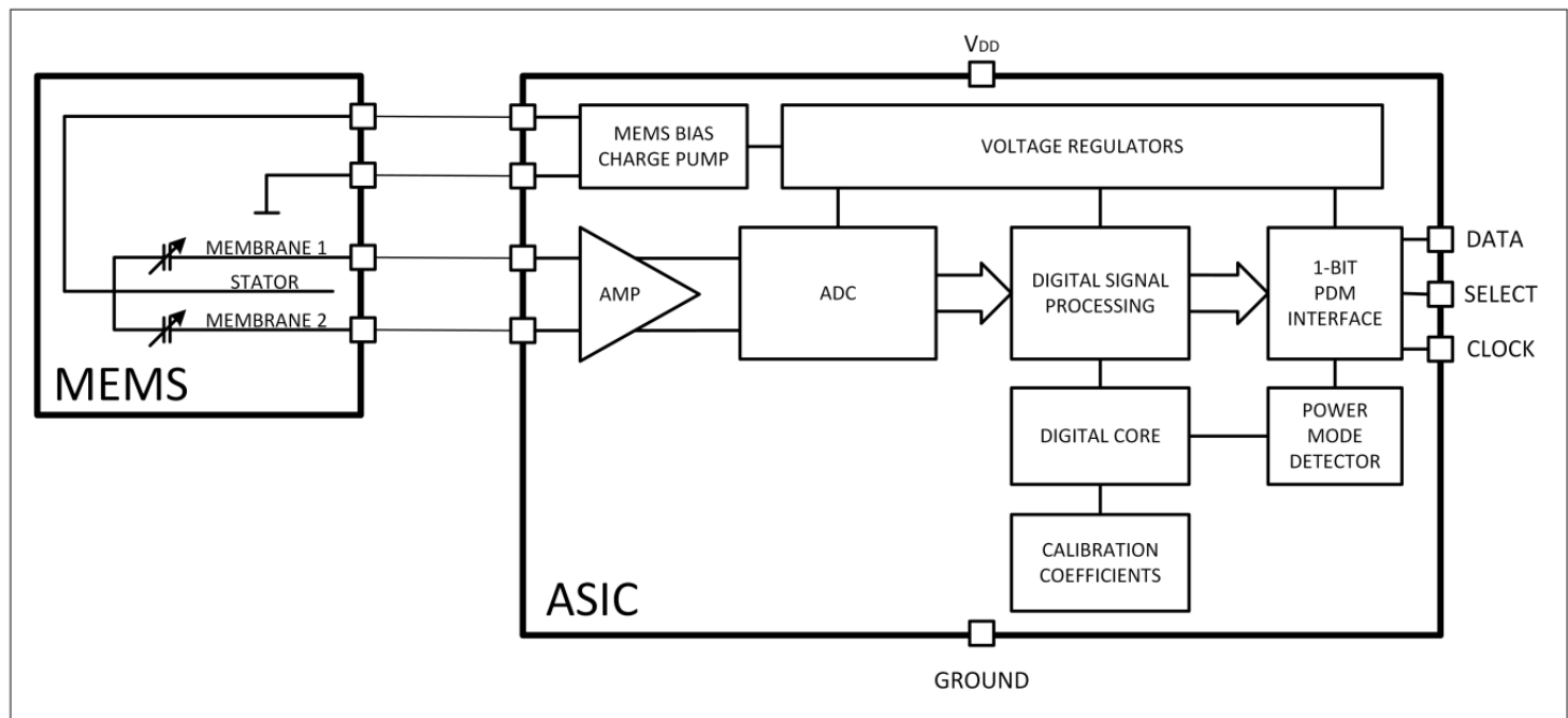
图 1 框图
