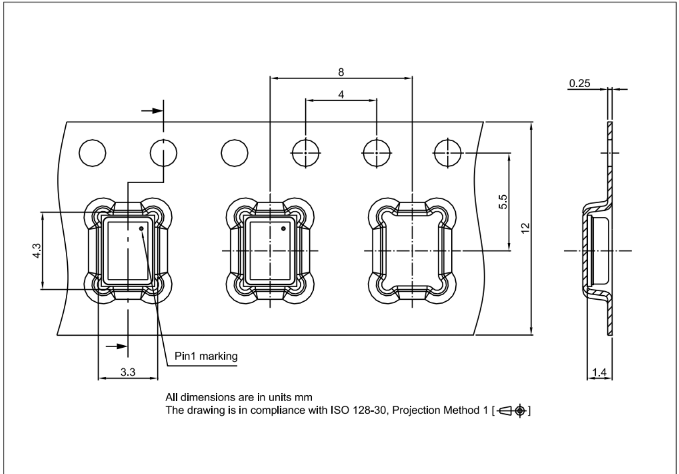
图14 IM72D128V01卷带包装信息
