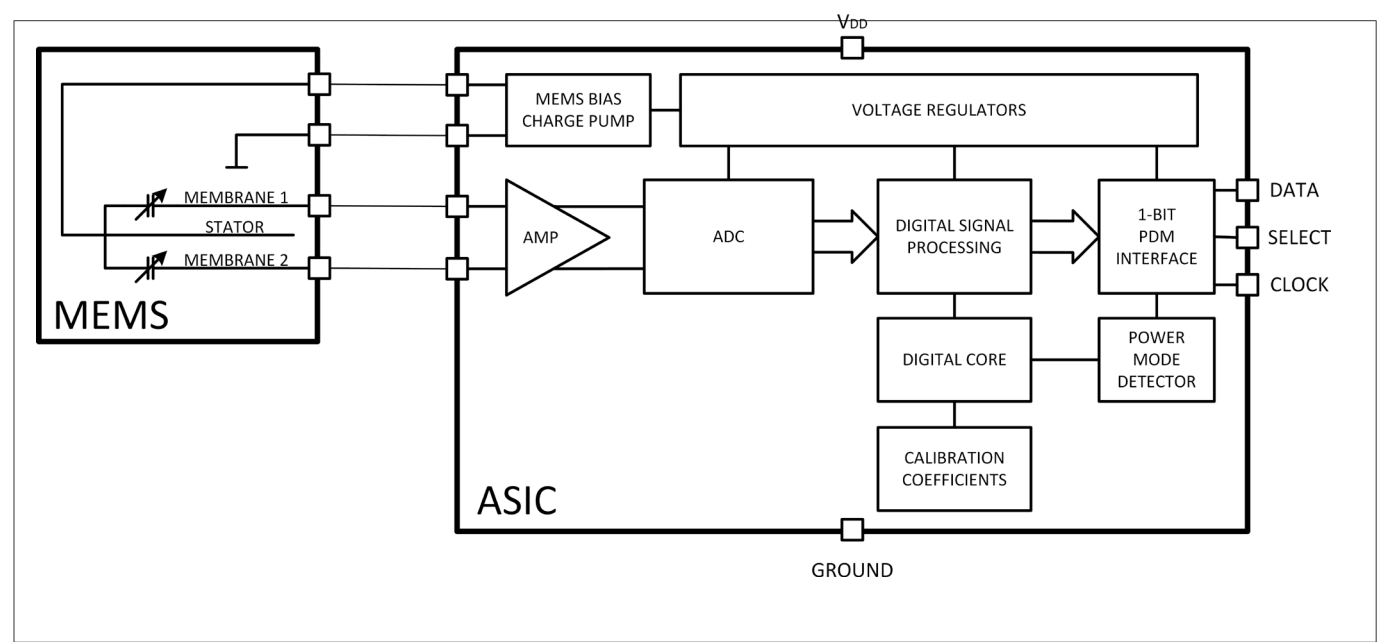
图 1 框图
