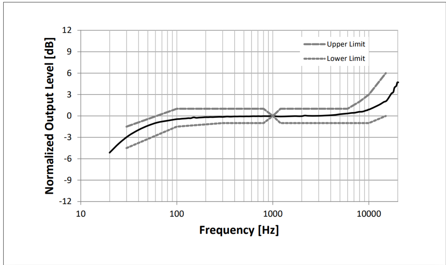
图10 IM70D122V01自由场频率响应
