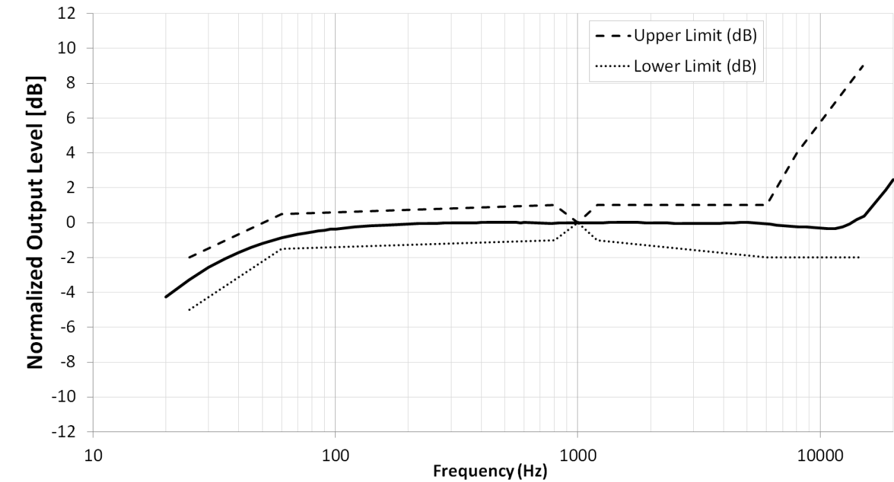
图8 IM69D120自由场频率响应
