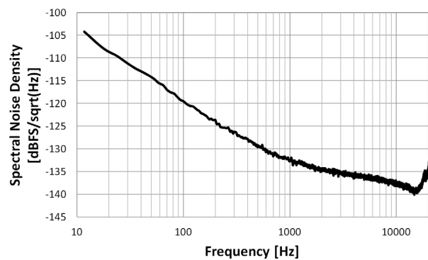
图 7 典型本底噪声（未加权）
