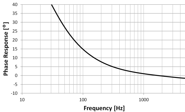
图 4 典型相位响应与频率的关系
