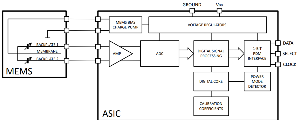
图1 IM69D120框图
