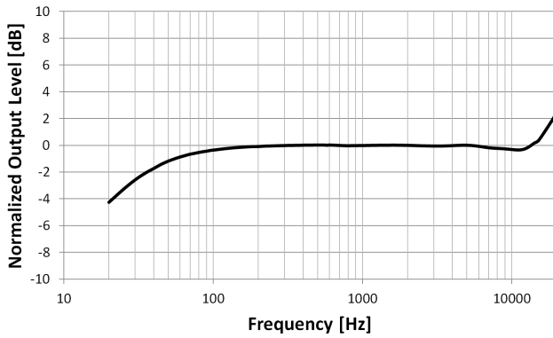
图 2 典型的自由场频率响应
