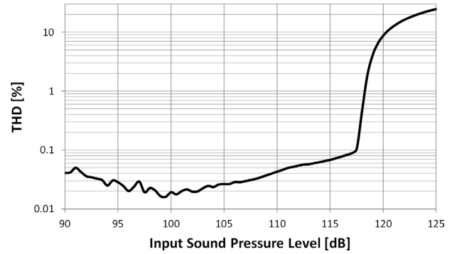
图 3 典型的 THD 与 SPL
