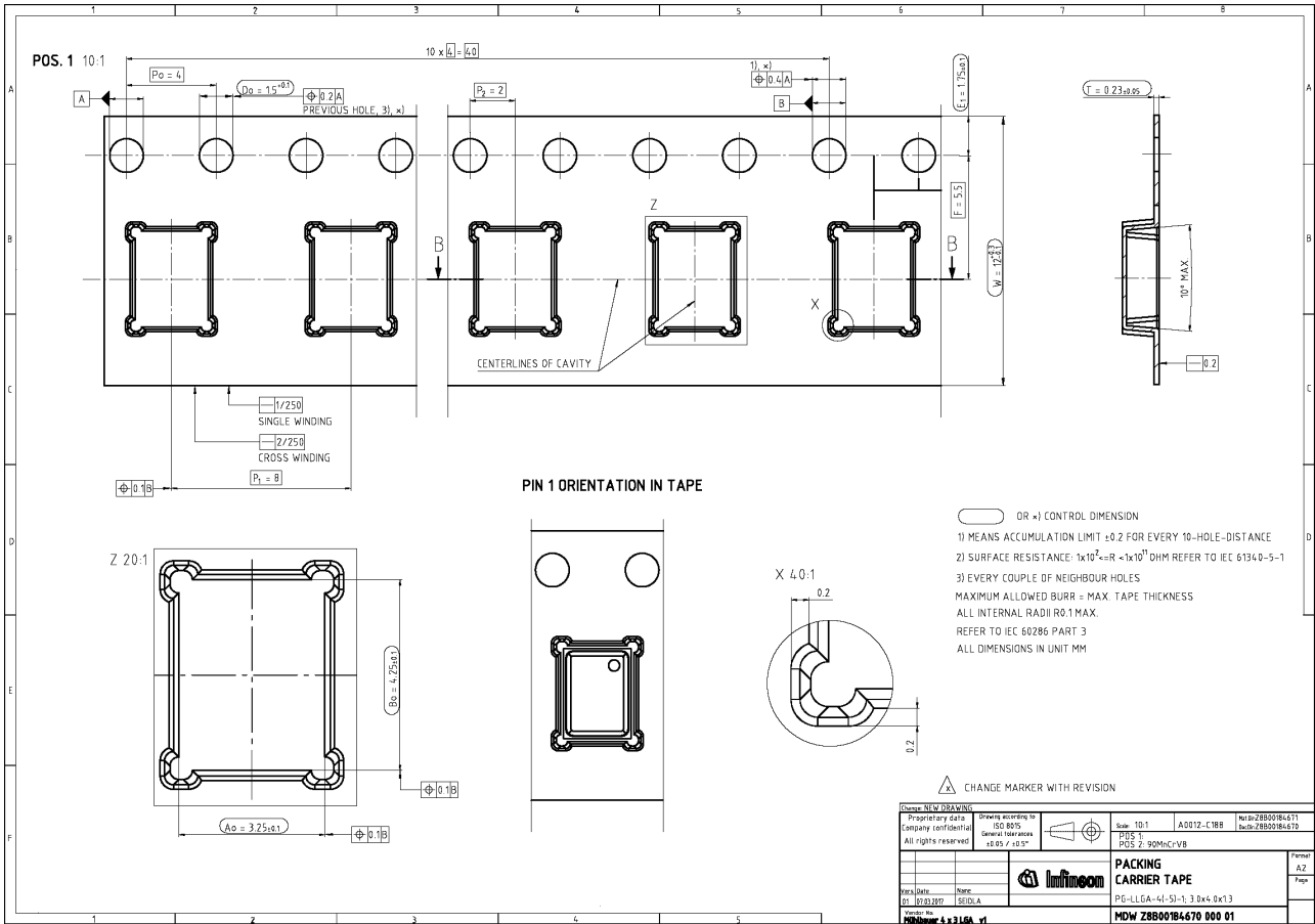
图 13 IM69D120 磁带尺寸
