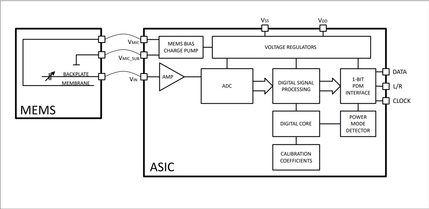
图 1 框图
