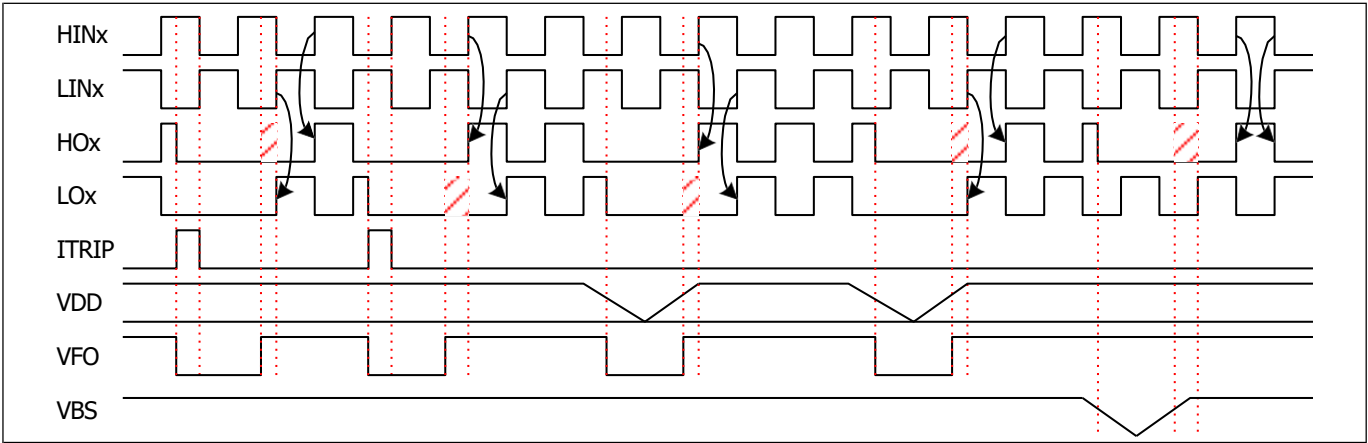
图10 休眠功能时序图
