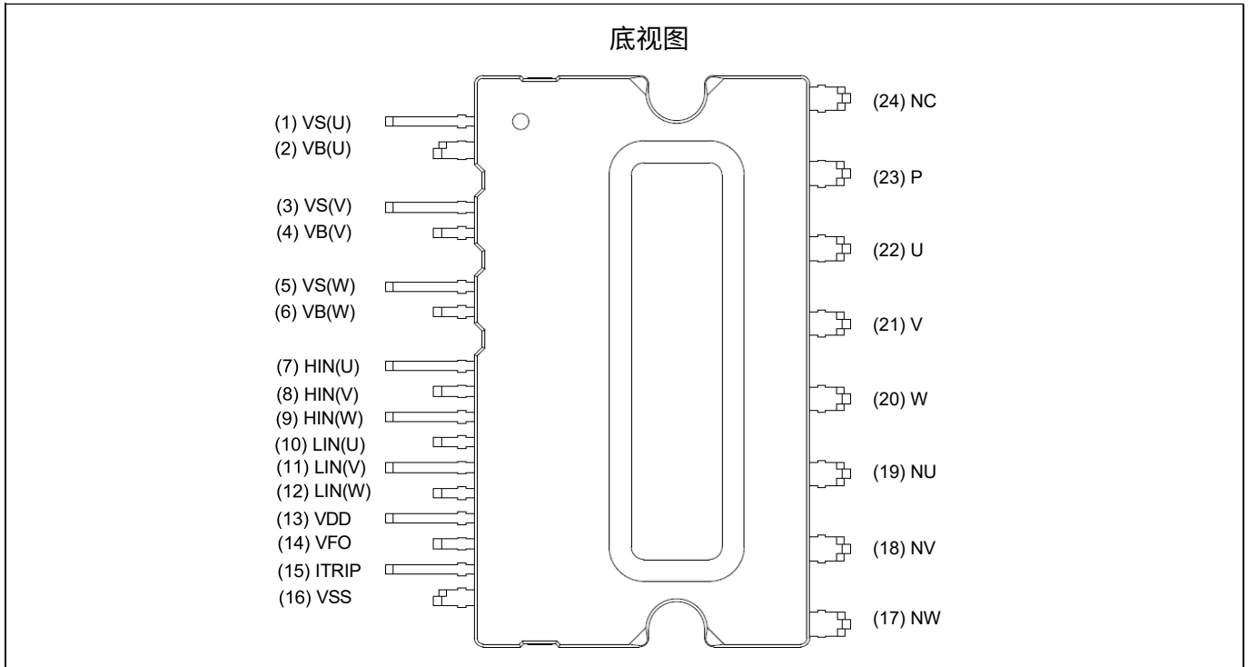
图 2 引脚配置
