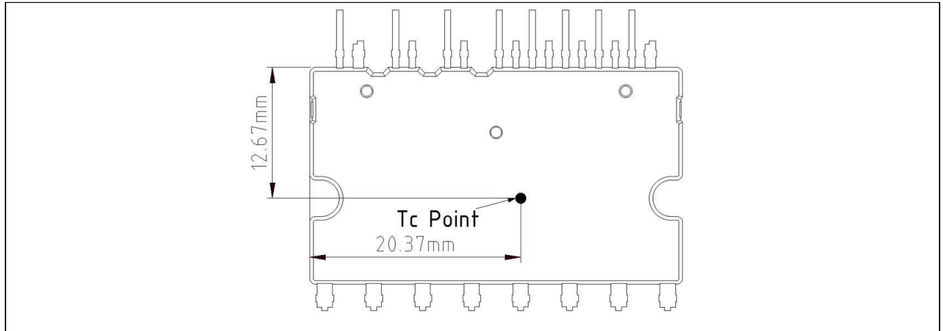
图7 T_c 测量点 1
