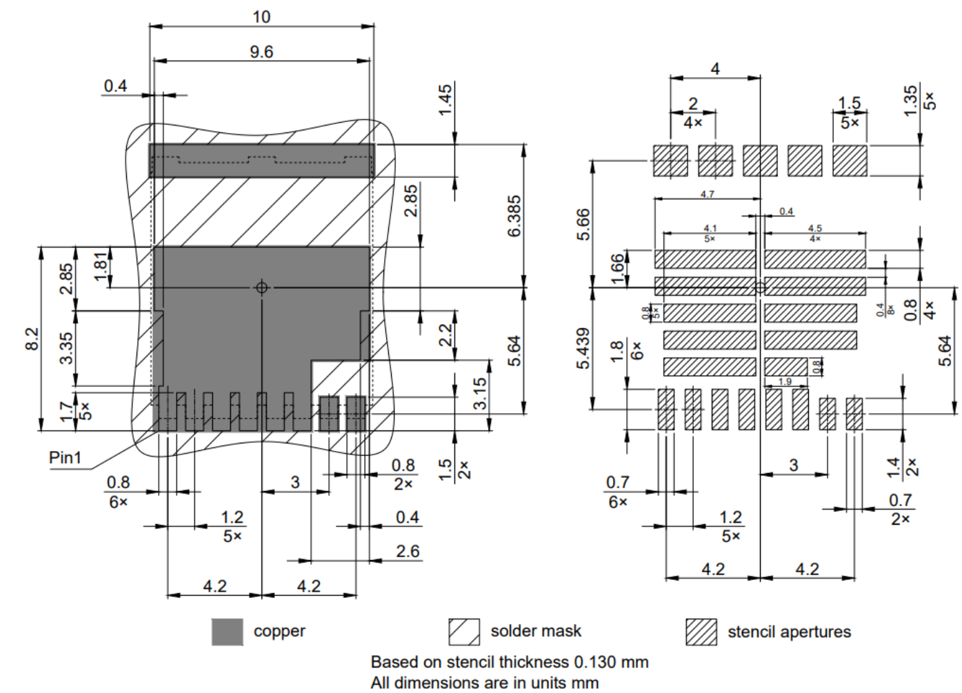
图 2 PG-HSOF-8 封装图，尺寸单位为毫米
