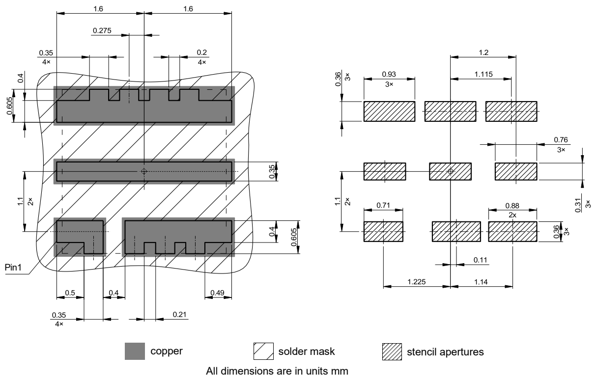
图 2 PG-VSON-4 封装图，尺寸单位为毫米
