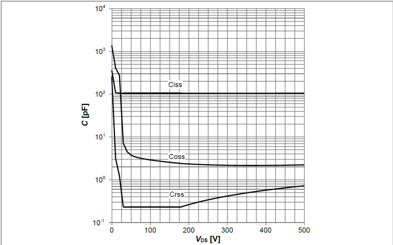
图 30 ICE5GR4780AG 的典型 CoolMOS™ 电容 ( C=f(V_{DS}) ; V_{GS}=0\text{ V} ; f=250\text{ kHz} )
