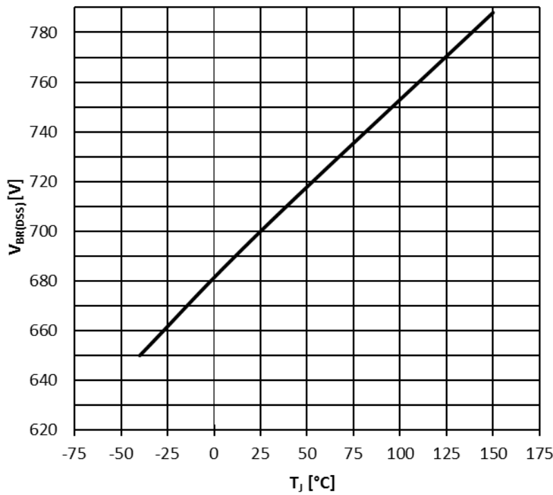
图 27 ICE5xRxx70AG 的漏源击穿电压; V_{BR(DSS)}=f(T_J) , I_D=1\text{ mA}
