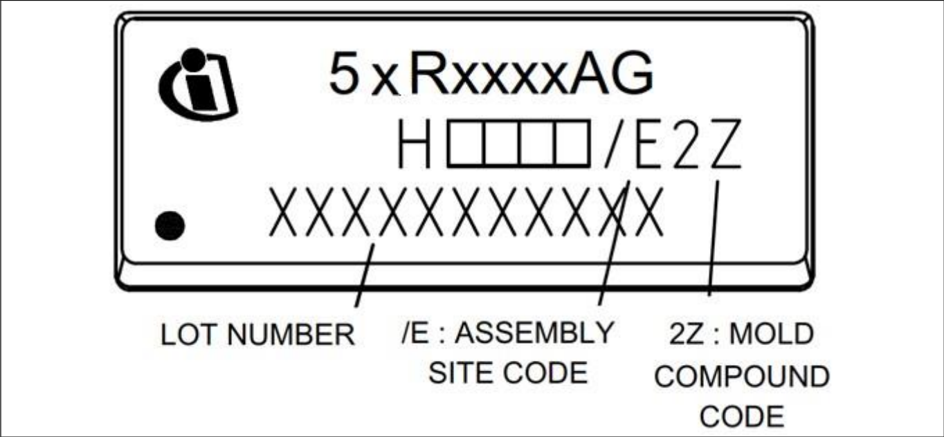
图 40 PG-DSO-12 标记
