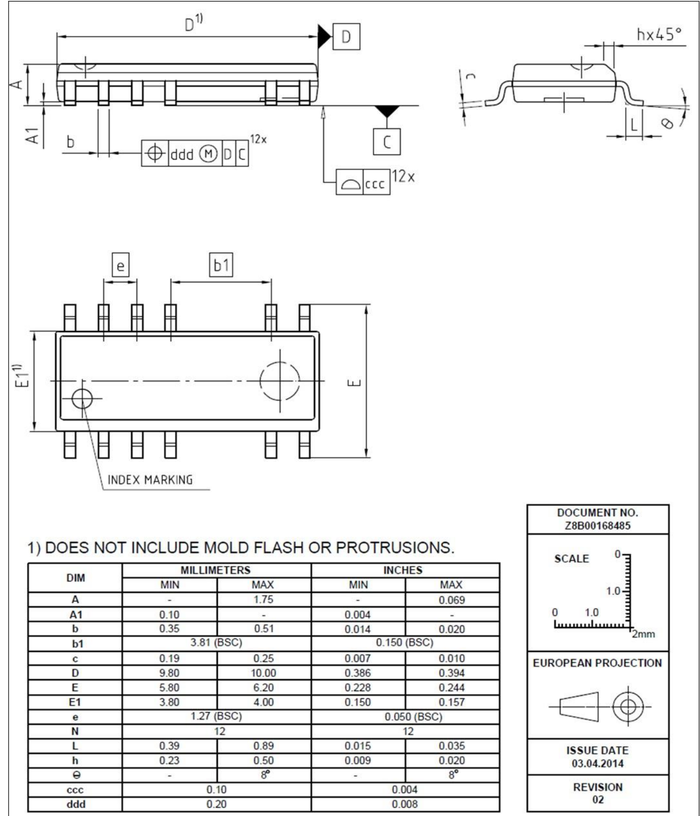
图 39 PG-DSO-12
