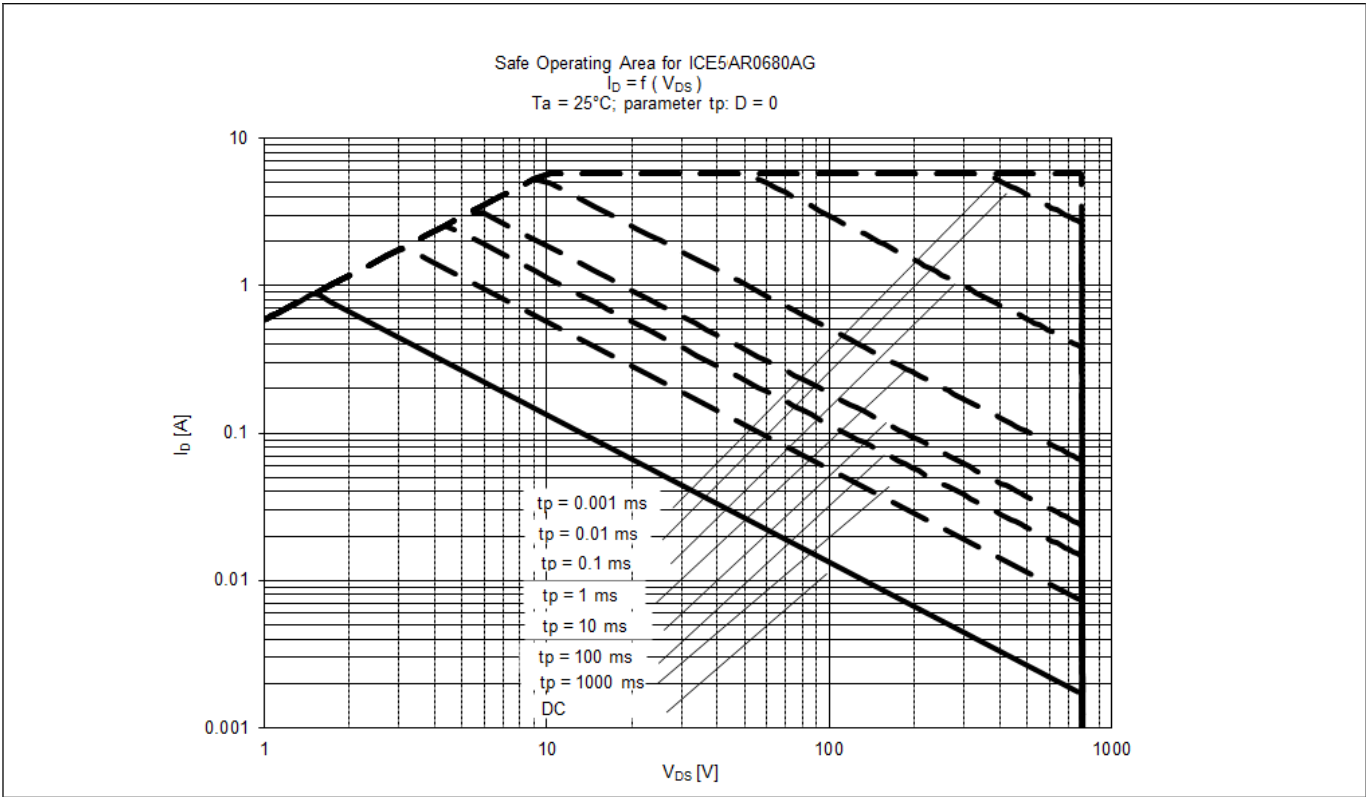
图 21 ICE5AR0680AG 的安全工作(SOA) 曲线
