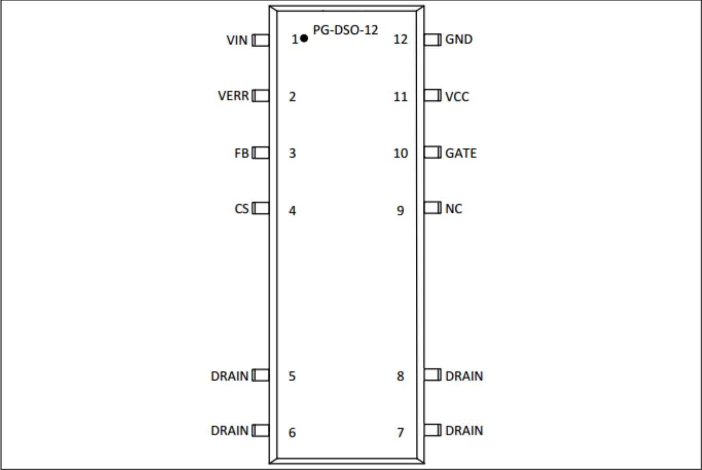
图 3 引脚配置
