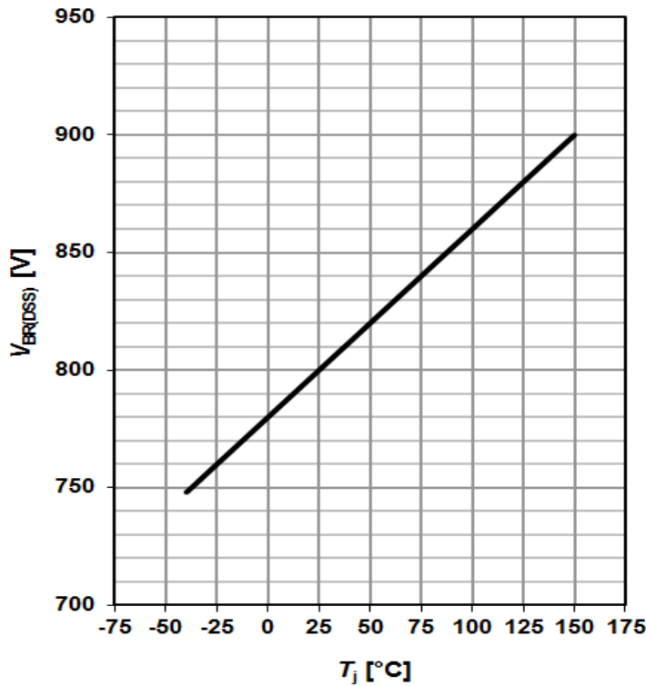
图 28 ICE5xRxx80AG 的漏源击穿电压; V_{BR(DSS)}=f(T_J) , I_D=1\text{ mA}
