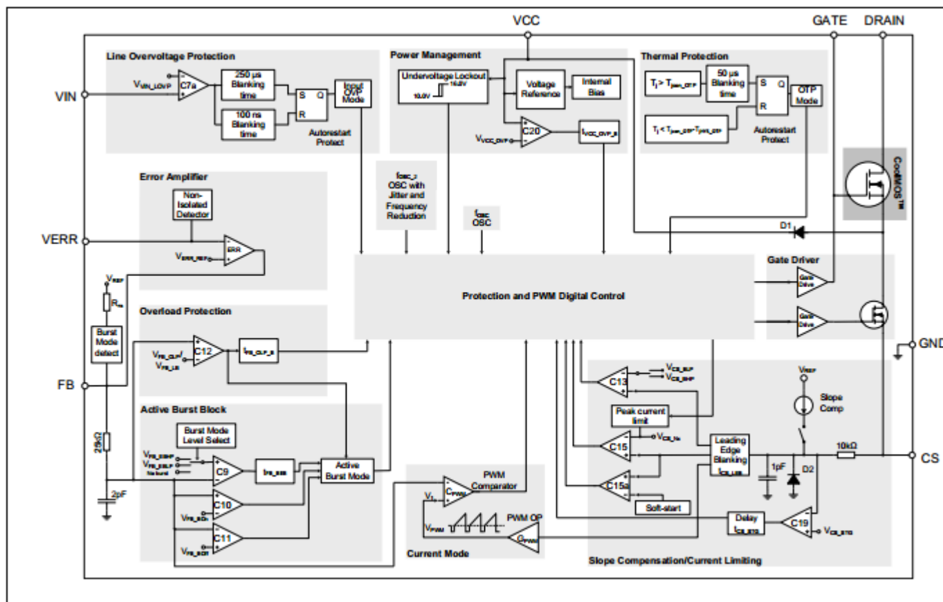
图 4 示例框图
