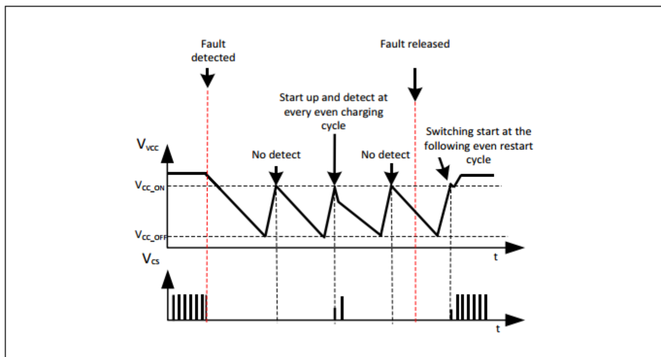
图 16 跳过奇数式自动重启
