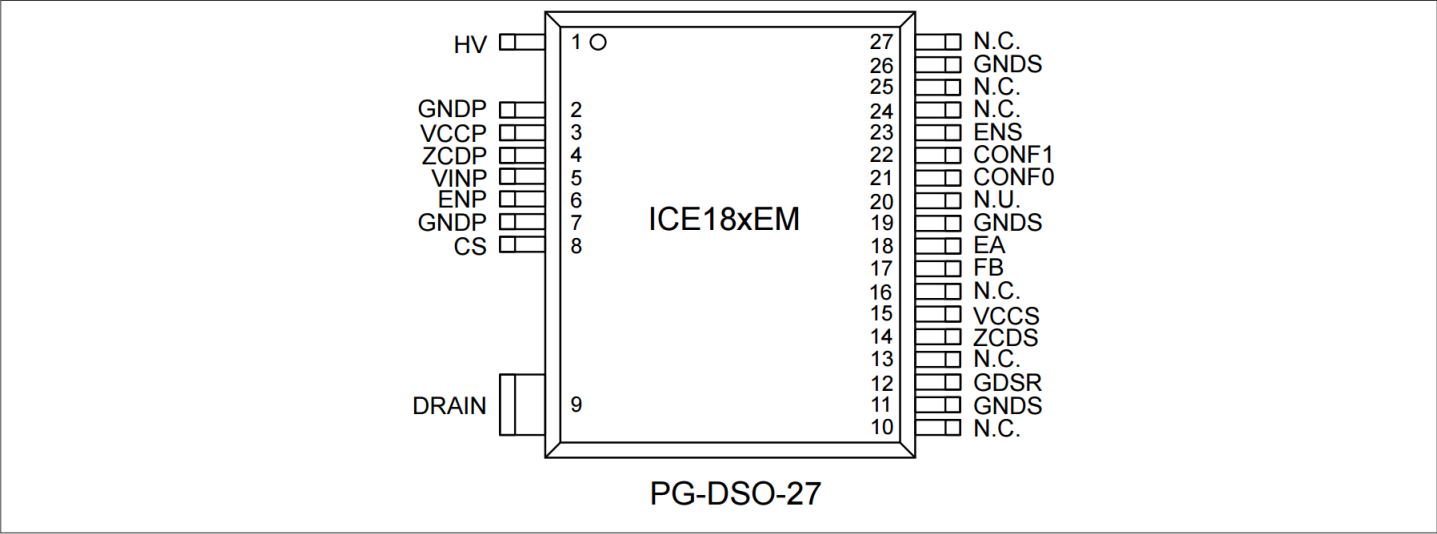
图 1 引脚配置
