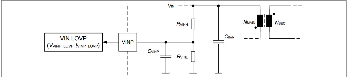
图 4 VINP 引脚检测
