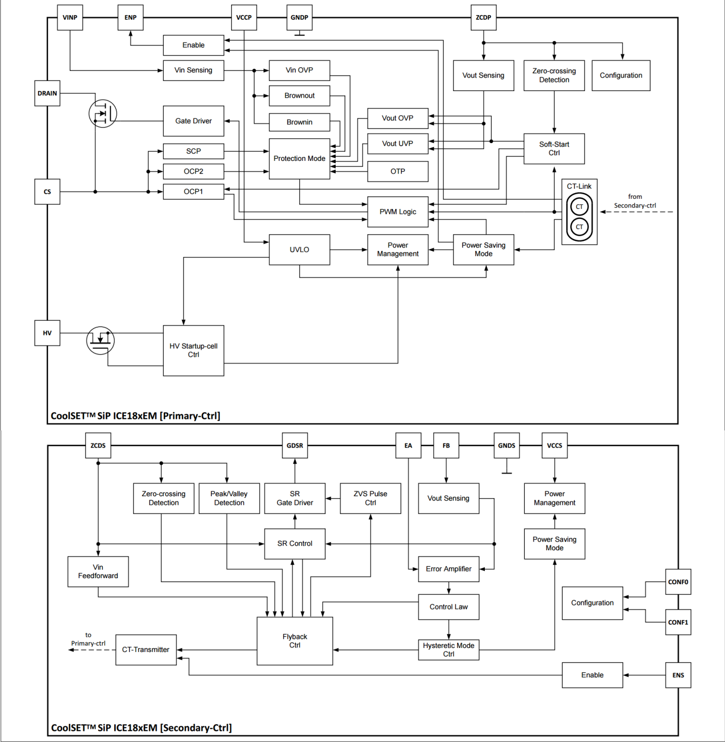
图 2 框图 CoolSET™ SiP ICE18xEM
