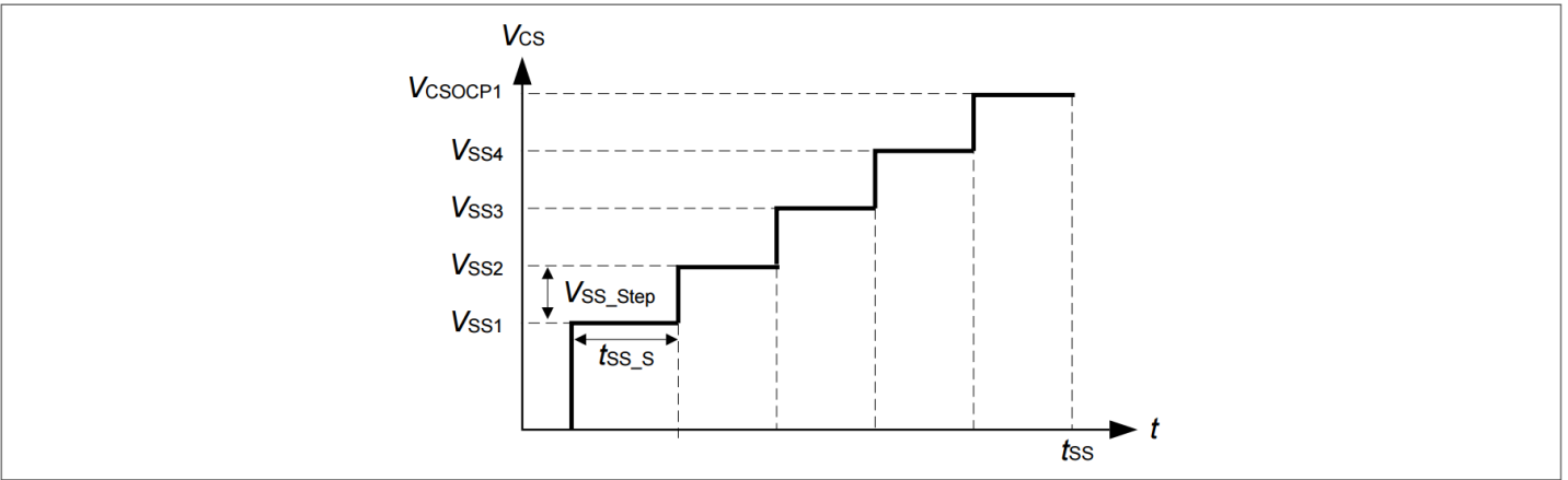
图 7 软启动期间的最大电流检测电压
