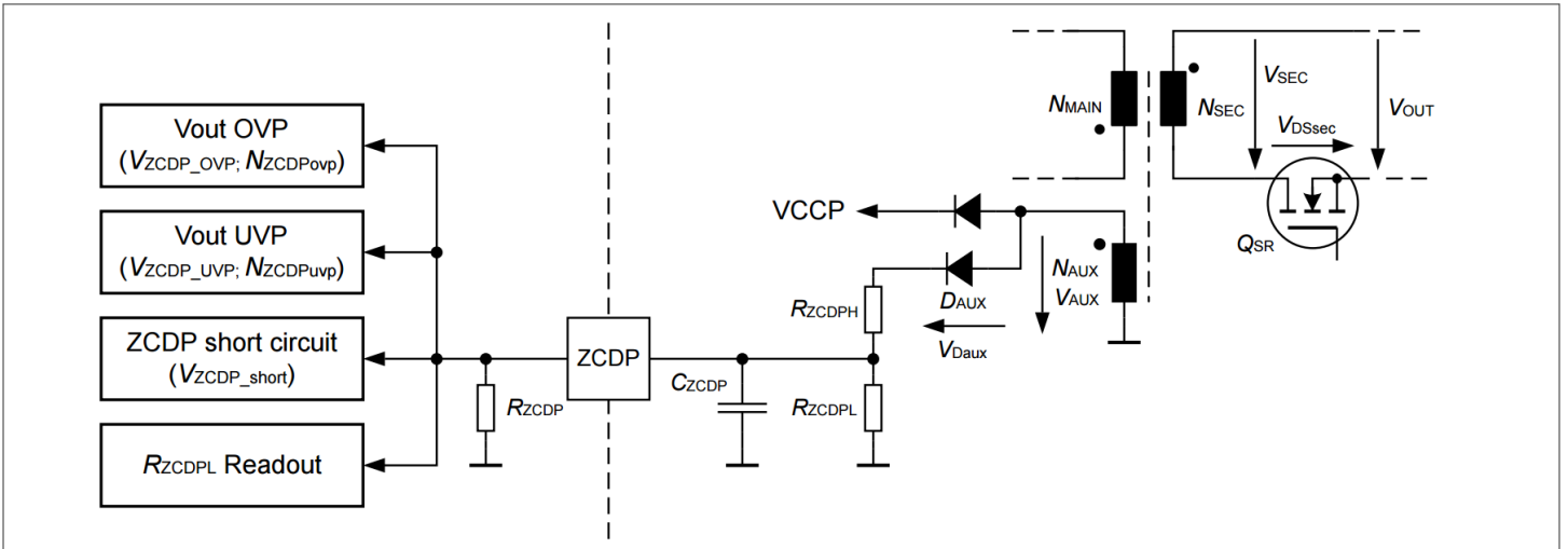
图 6 初级侧 ZCDP 引脚检测
