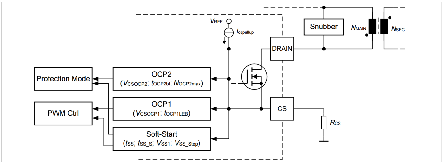
图 5 CS 引脚的初级侧电流检测
