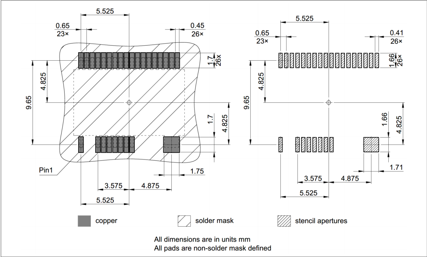
图 11 封装
