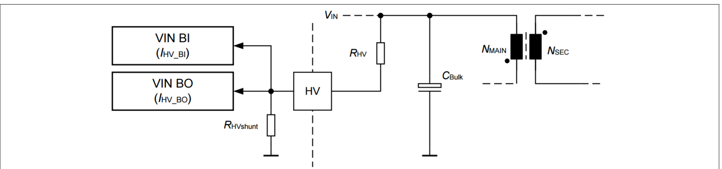
图 3 用于 brownin/brownout 保护的高压引脚检测
