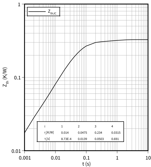
過渡熱インピーダンス, Diode、ブレーキチョッパー Z_{th} = f(t)
