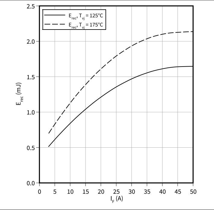
开关损耗（典型), 二极管, 逆变器
