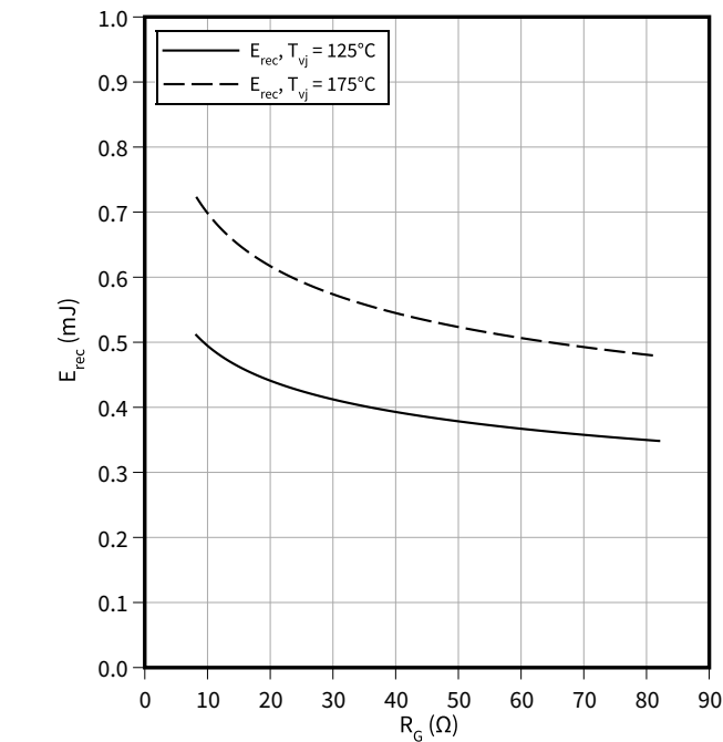
开关损耗（典型），二极管,逆变器 E_{rec} = f(R_G) I_F = 10 A, V_{CC} = 600 V
