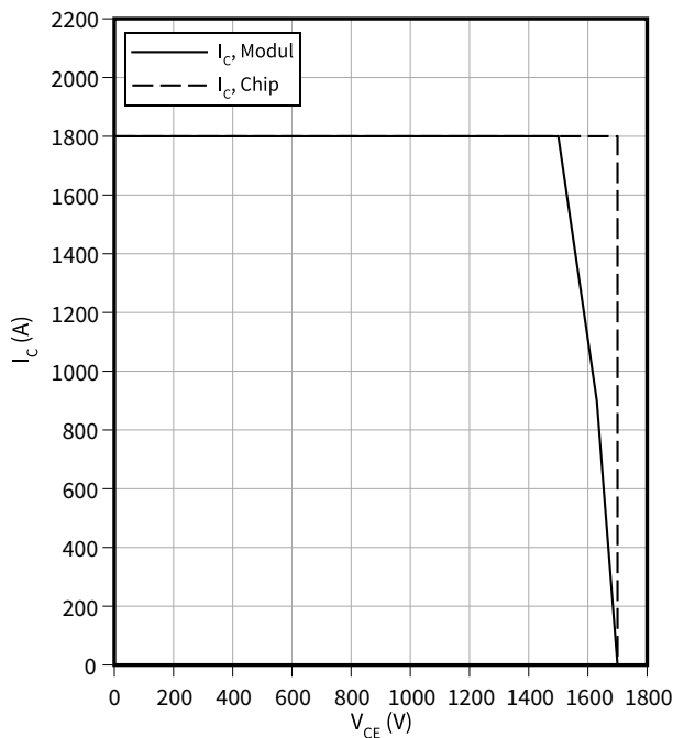
逆バイアス安全動作領域 (RBSOA), IGBT- インバータ I_C = f(V_{CE}) R_{Goff} = 3 \Omega , V_{GE} = \pm 15 \text{ V} , T_{vj} = 175 \text{ °C}
