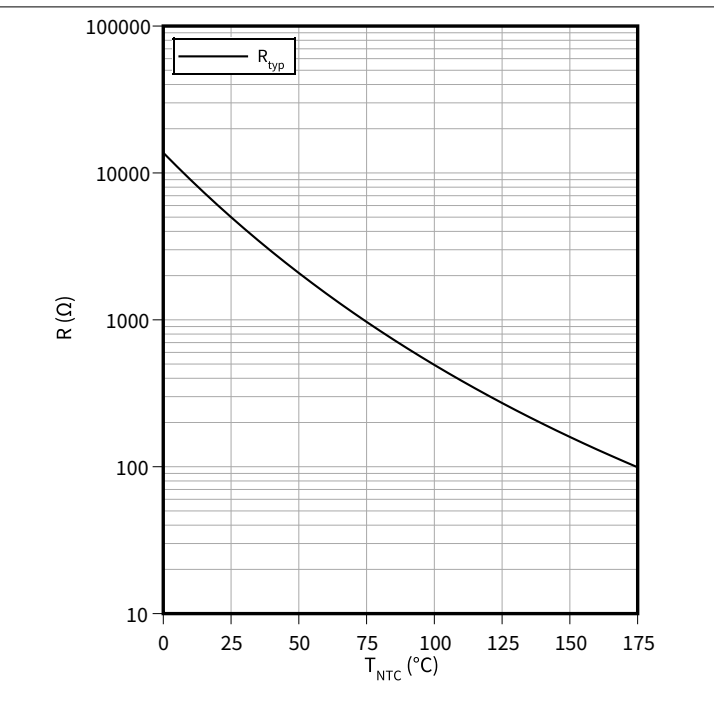
温度特性，负温度系数热敏电阻
