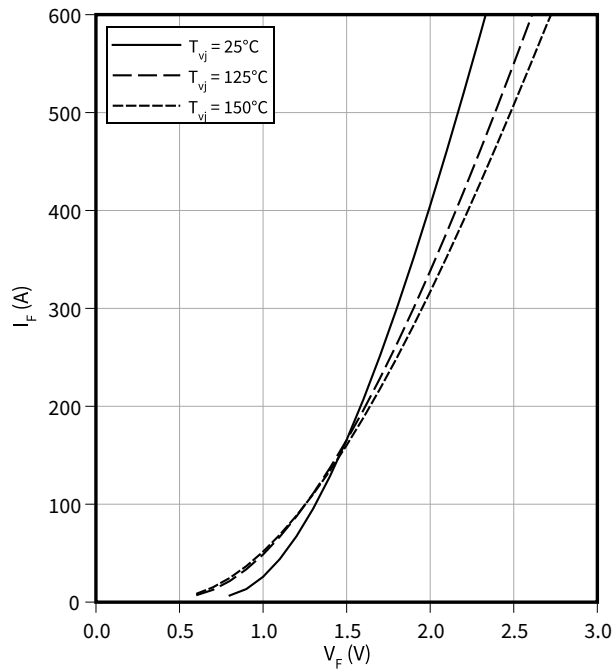
順電圧特性 (typical), Diode、リバース
