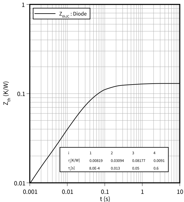
過渡熱インピーダンス, Diode、ブレーキチョッパー
