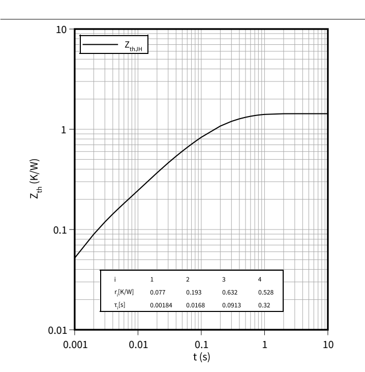
過渡熱インピーダンス, Diode、整流器 Z_{th} = f(t)
