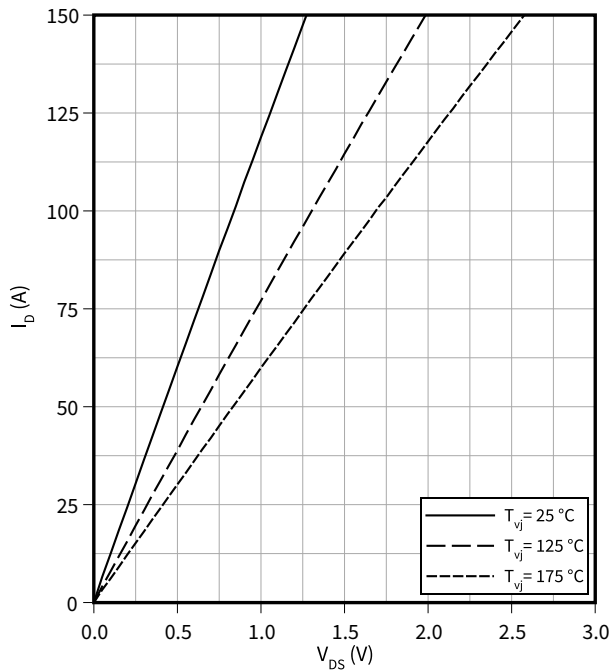
出力特性 (typical), MOSFET, T1-T4
