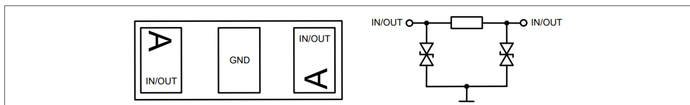
图1 引脚配置及原理图
