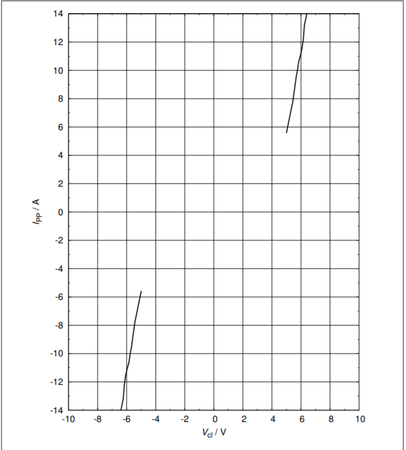
图10 钳位电压（浪涌）： I_{PP} = f(V_{cl}) ，基于IEC61000-4-5
