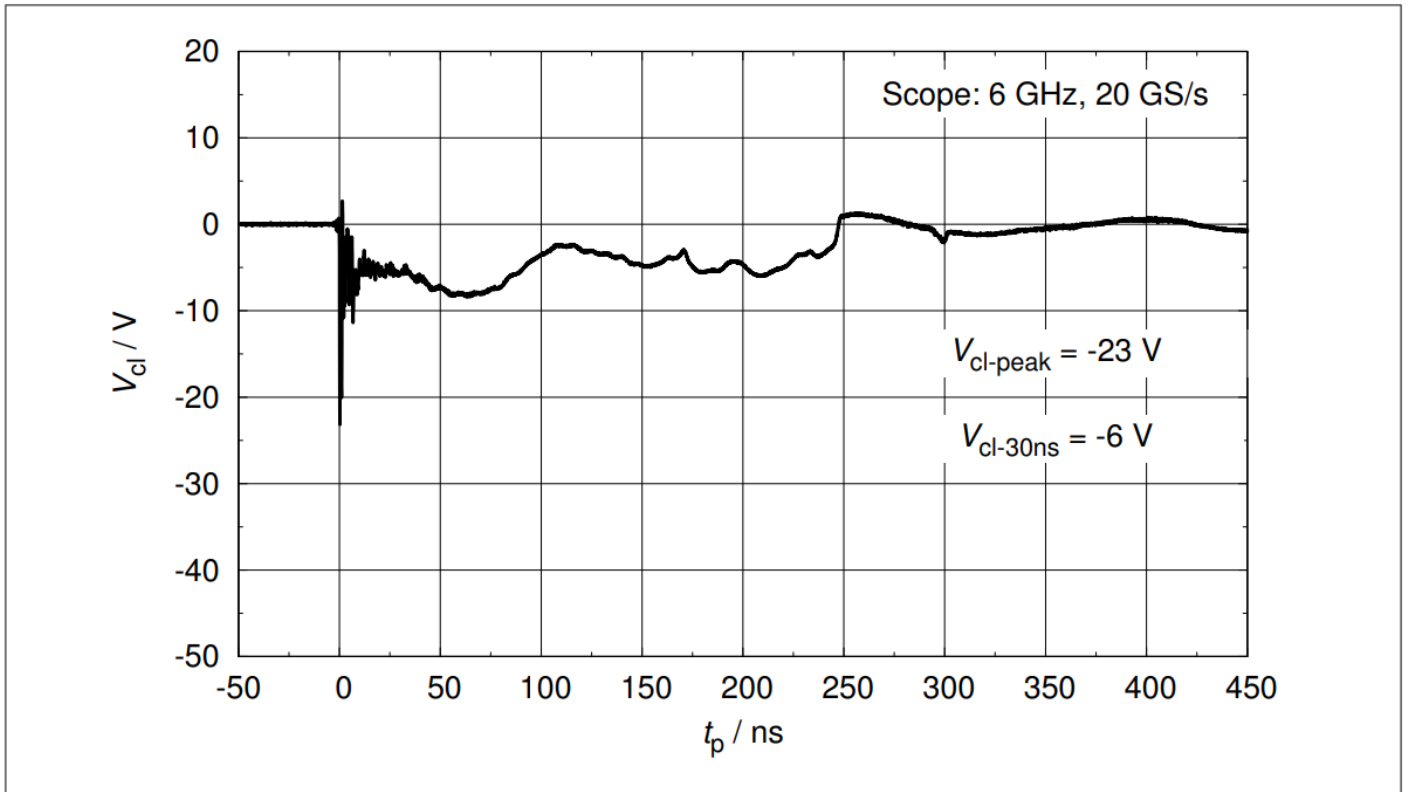
图6 钳位电压 (ESD) : V_{cl}=f(t_p) , 8kV负脉冲基于IEC61000-4-2
