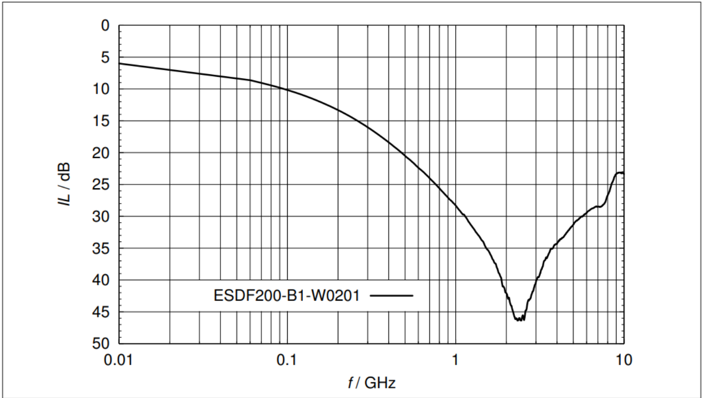
图11 插入损耗: IL = f(f) , 在50 Ω系统中测量
