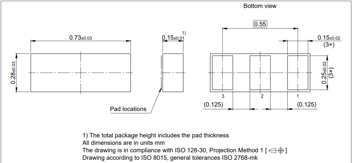
图12 WLL-3-2封装
