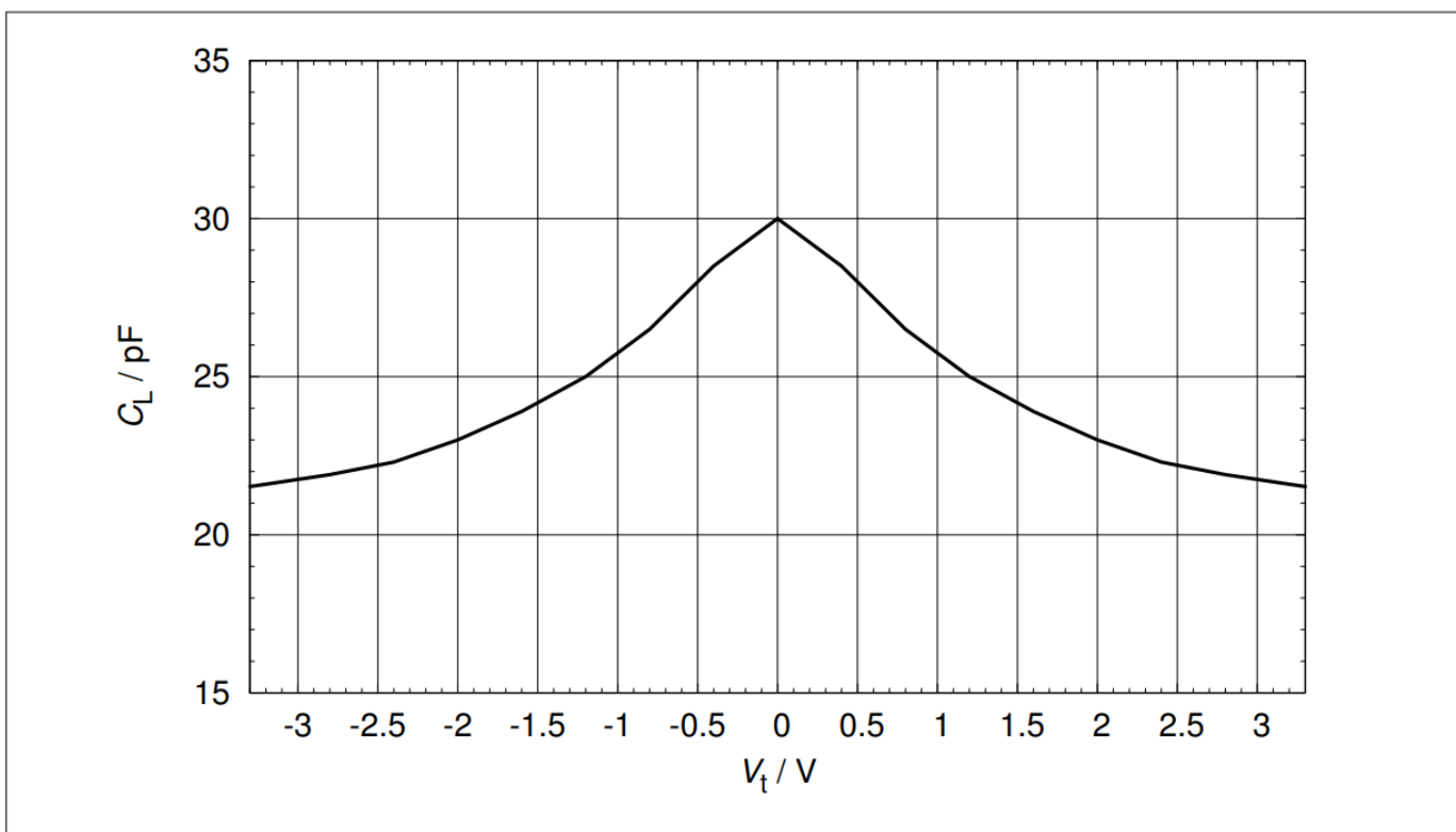
图4 线路电容： C_L = f(V_t) , f = 1\text{ MHz}
