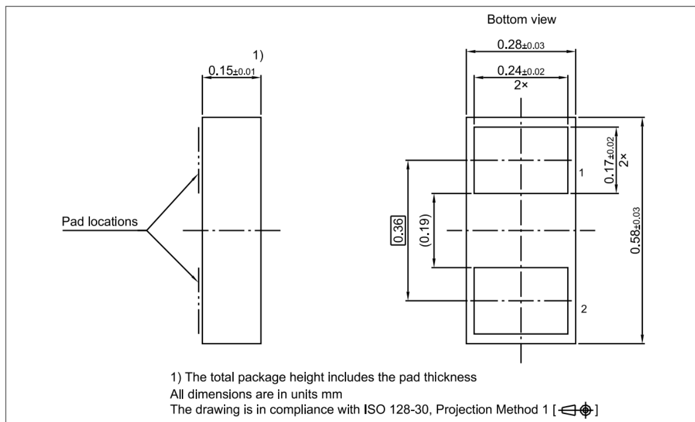
图12 WLL-2-3封装
