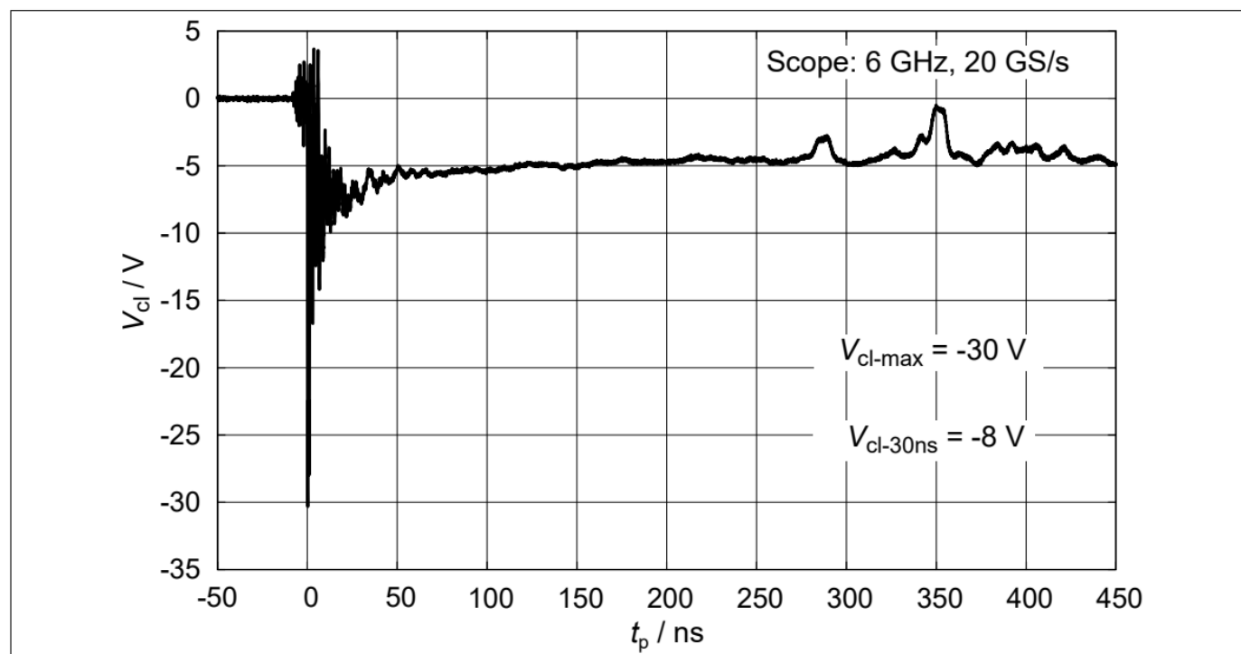
图8 钳位电压 (ESD) : V_{cl}=f(t_p) , 15kV负脉冲基于IEC61000-4-2
