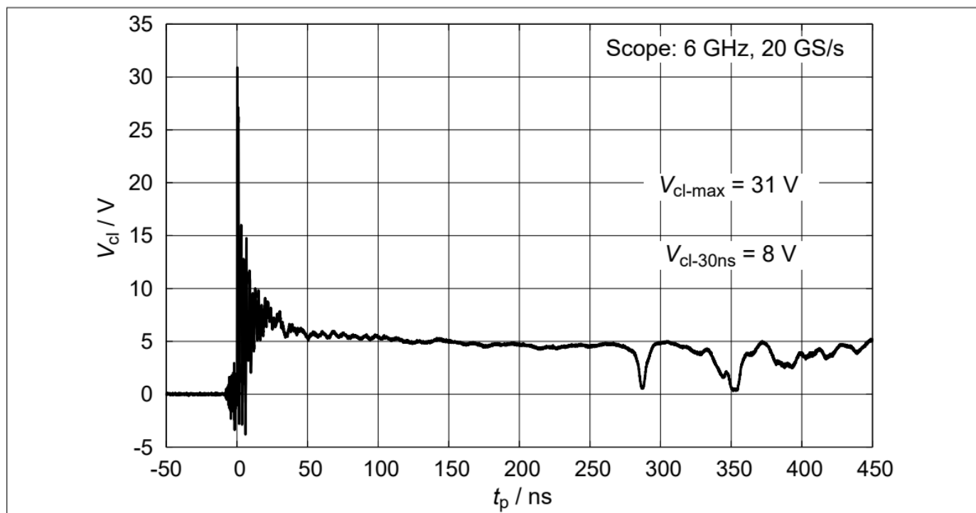
图7 钳位电压 (ESD) : V_{cl}=f(t_p) , 15kV正脉冲 , 基于IEC61000-4-2
