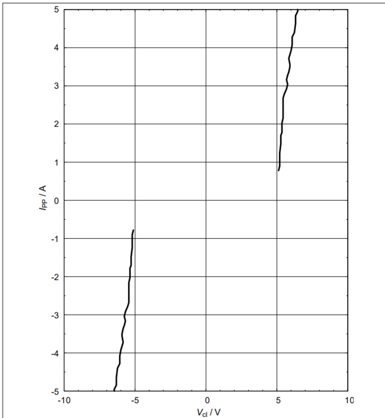
图10 钳位电压（浪涌）： I_{PP} = f(V_{CL}) ，基于IEC61000-4-5
