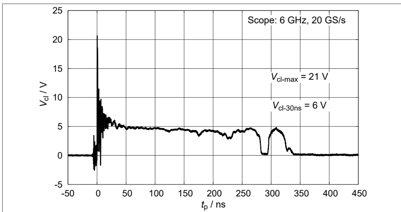
图5 钳位电压 (ESD) : V_{cl}=f(t_p) , 8kV正脉冲, 基于IEC61000-4-2
