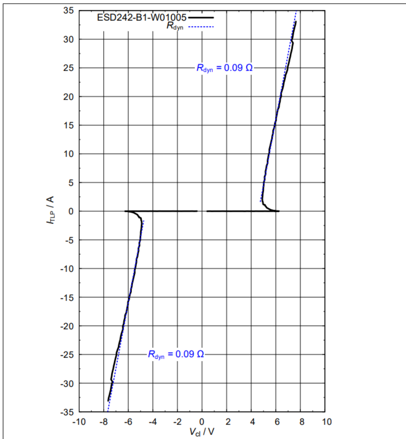
图9 钳位电压 (TLP) : I_{TLP} = f(V_{cl})
