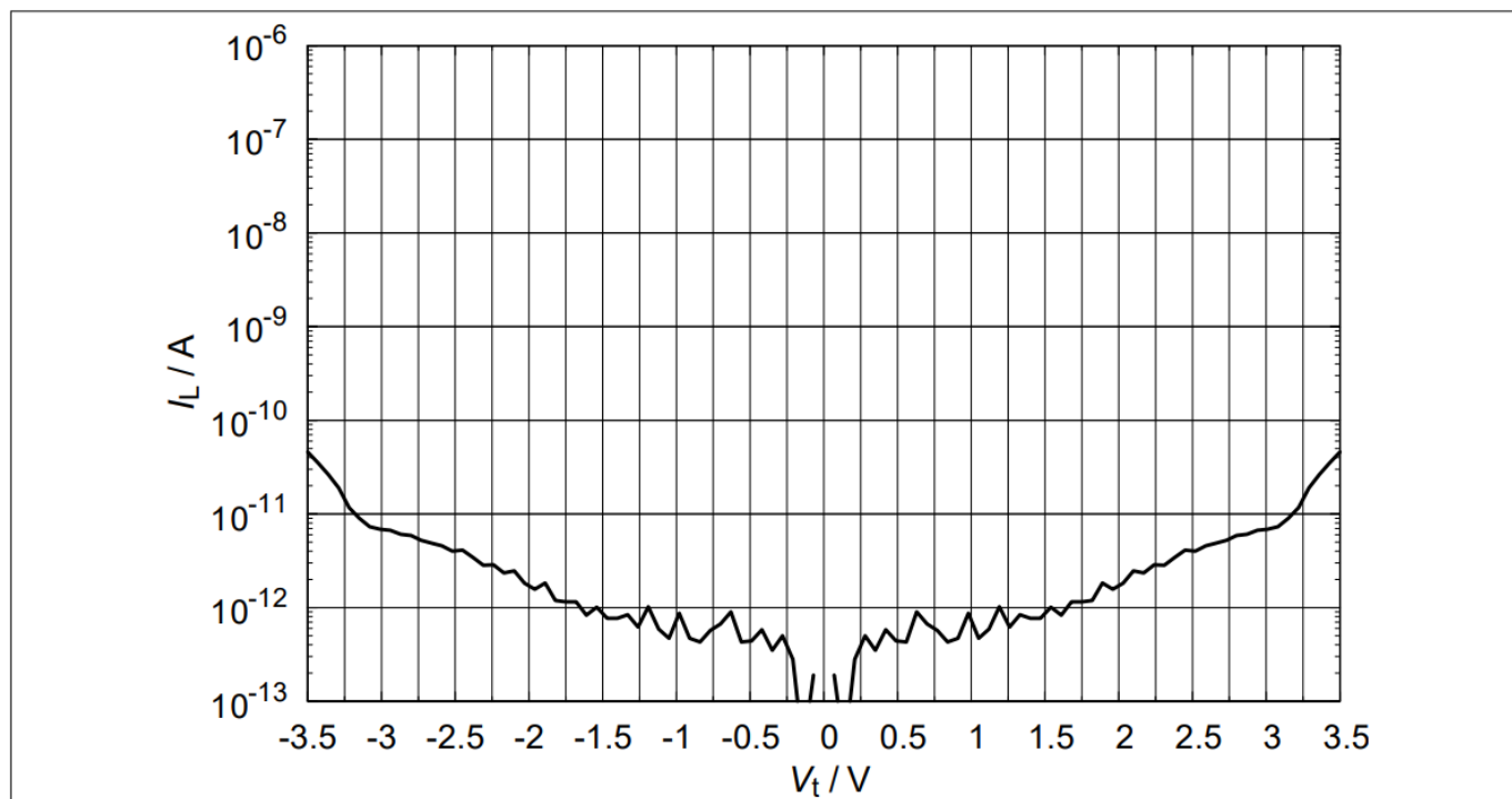
图3 漏电流： I_L = f(V_t)
