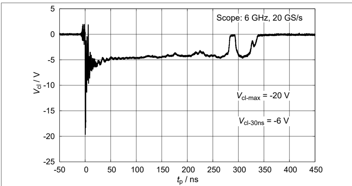
图6 钳位电压 (ESD) : V_{cl}=f(t_p) , 8kV负脉冲基于IEC61000-4-2
