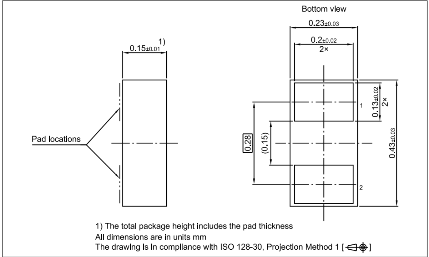
图12 WLL-2-2封装
