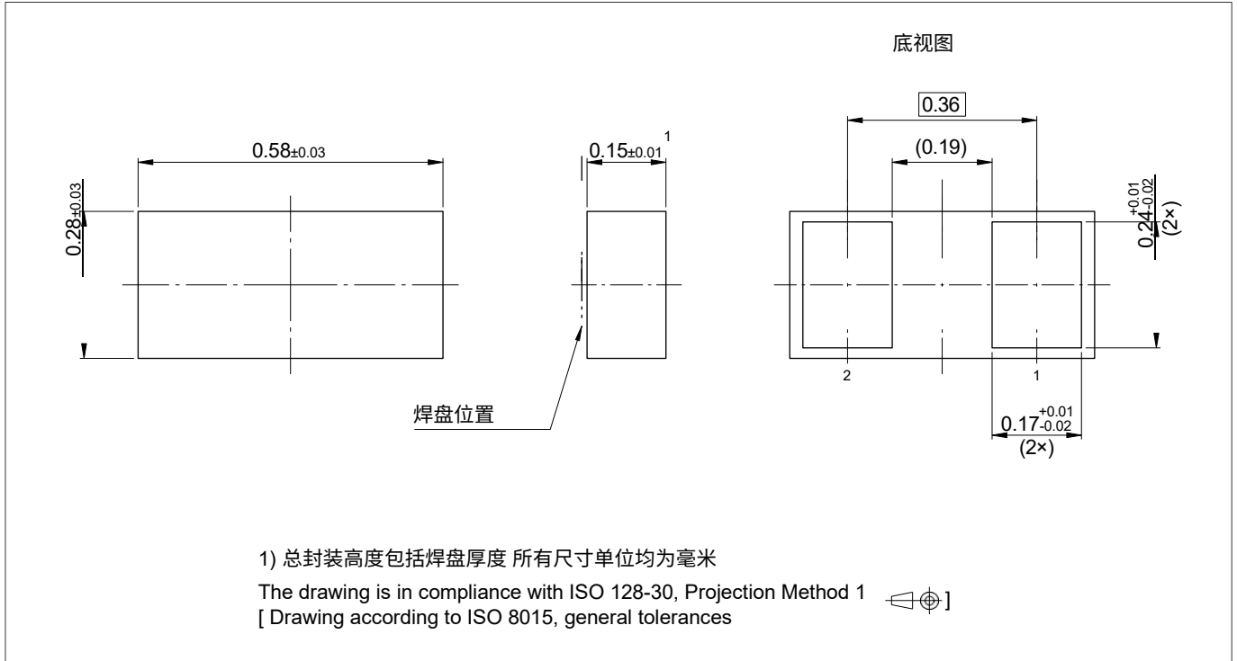
图12 WLL-2-3封装
