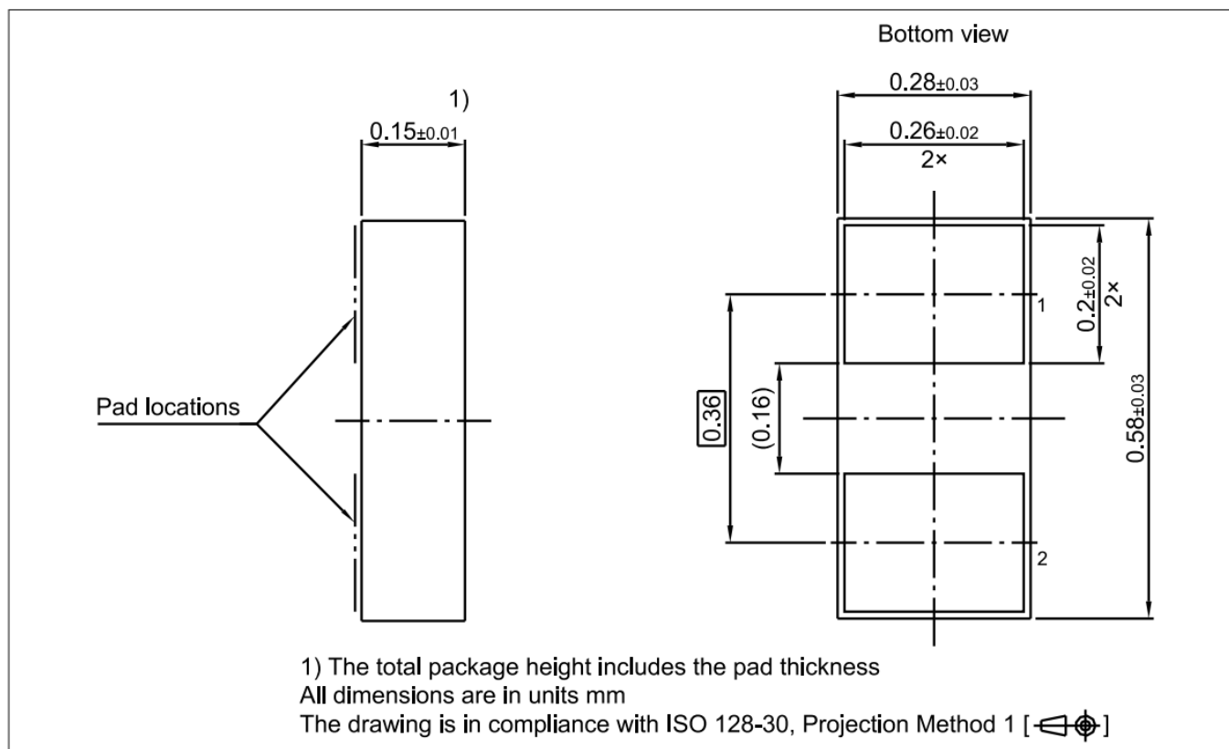
图12 WLL-2-1封装
