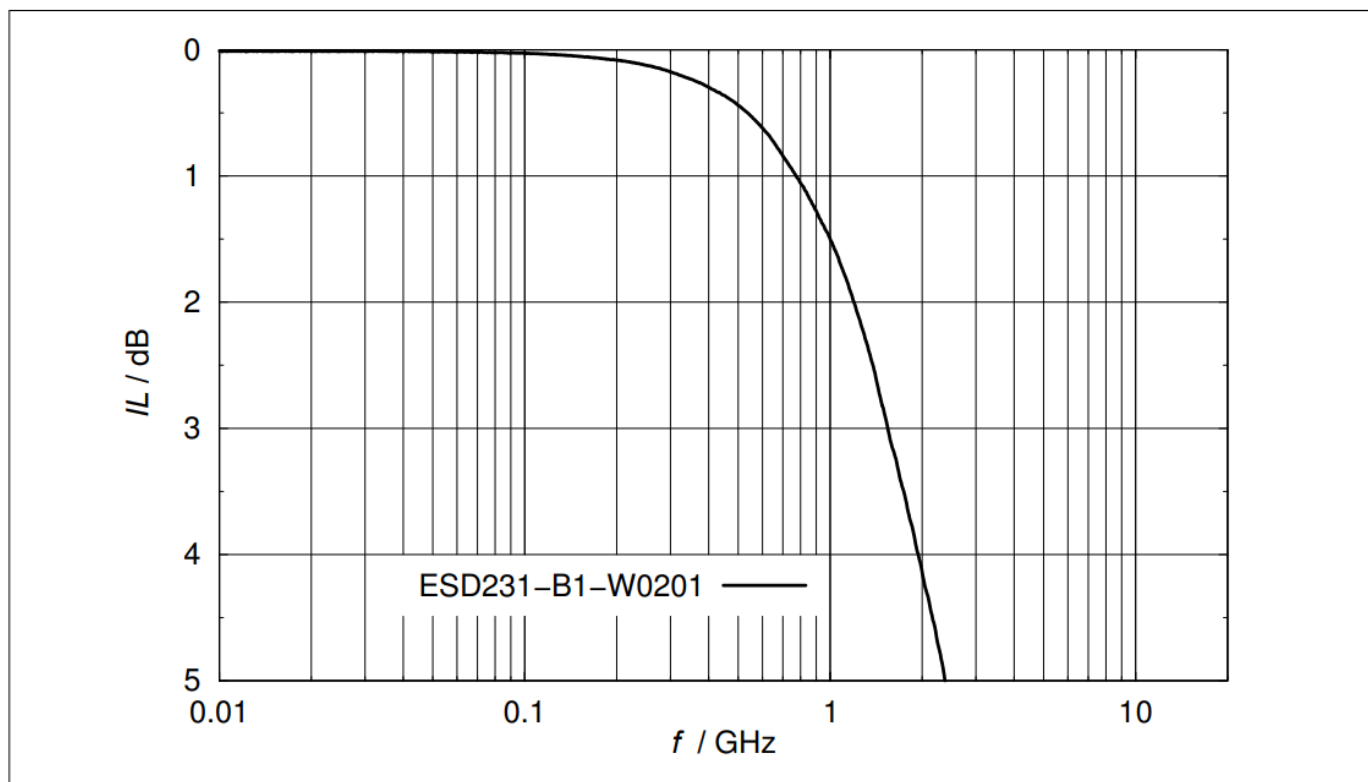
图11 50 \Omega 系统中插入损耗与频率的关系
