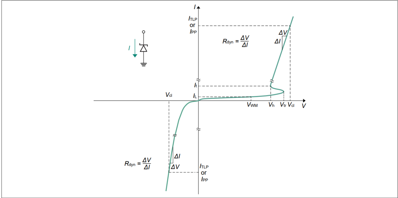
图2 I / V特性曲线
