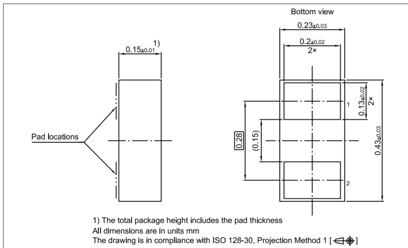
图12 WLL-2-7封装
