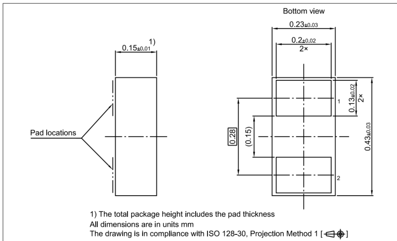
图13 WLL-2-2封装
