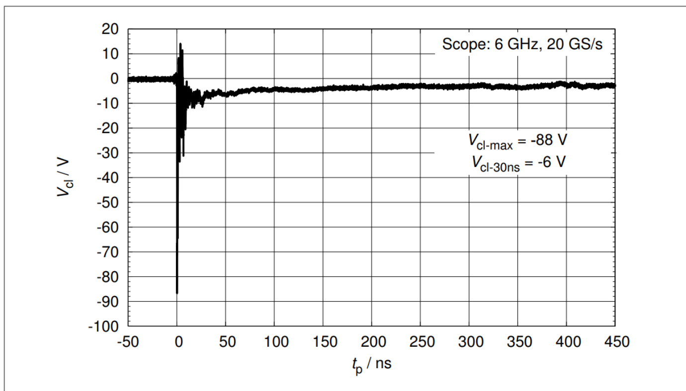
图8 钳位电压 (ESD) : V_{cl}(t_p) = f(t_p) , 15kV负脉冲基于IEC61000-4-2
