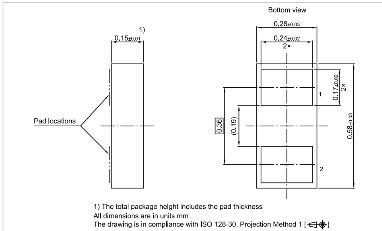
图13 WLL-2-3封装
