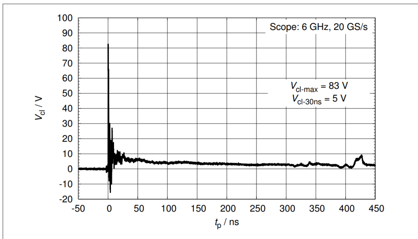
图7 钳位电压 (ESD) : V_{cl}(t_p) = f(t_p) , 15kV正脉冲, 基于IEC61000-4-2
