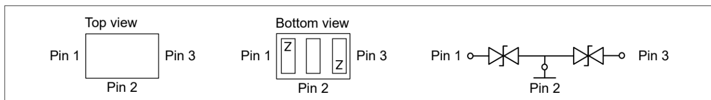
图1 引脚配置及原理图
