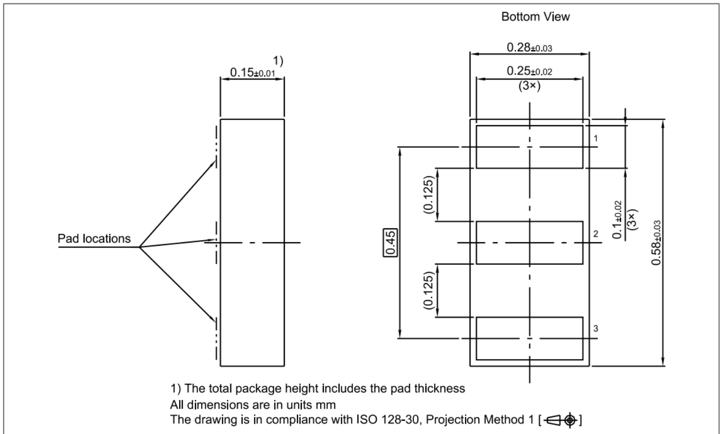
图13 WLL-3-1封装
