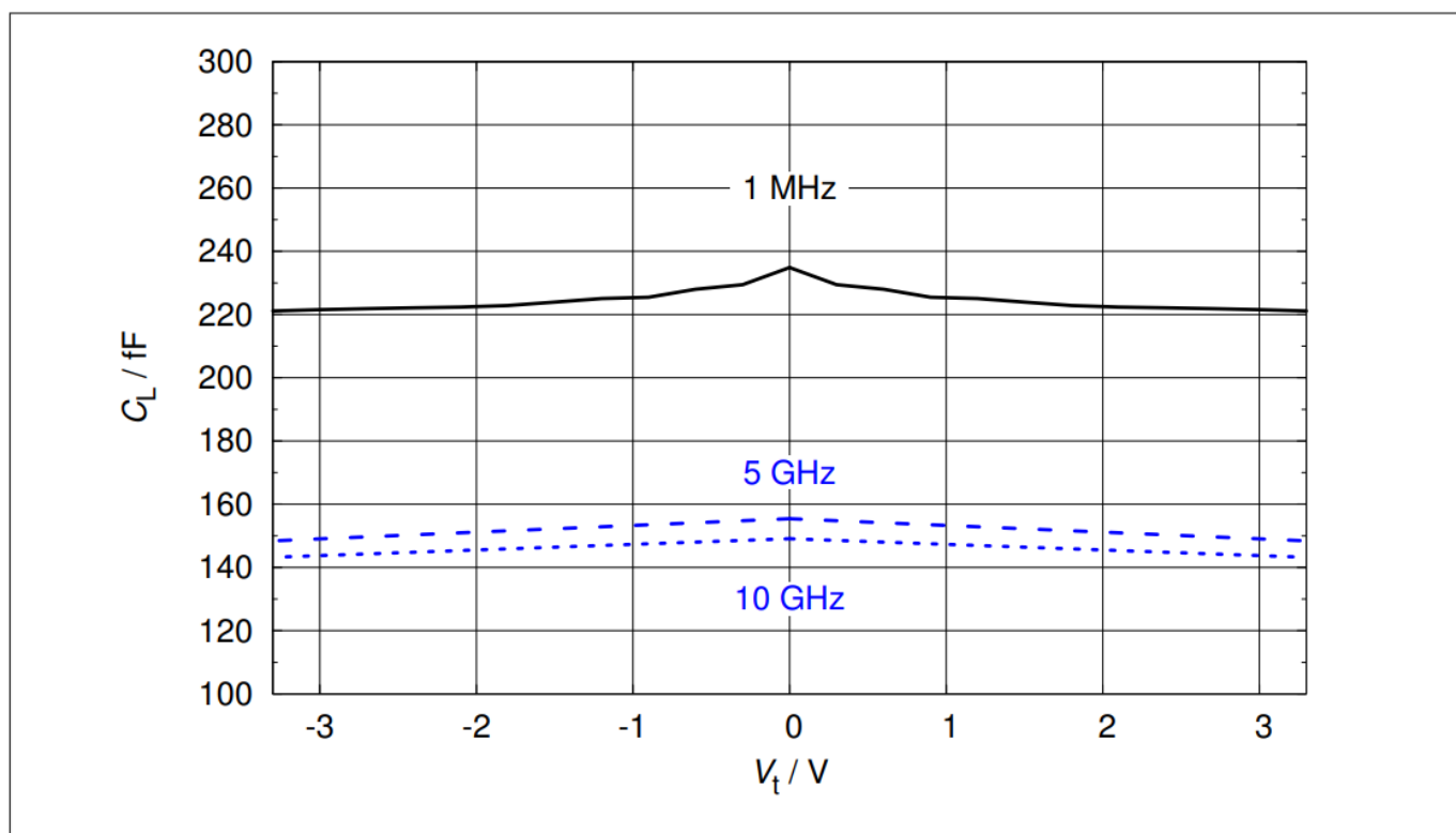
图4 线路电容： C_L = f(V_t) , f = 1\text{ MHz} 、 5\text{ GHz} 、 10\text{ GHz}
