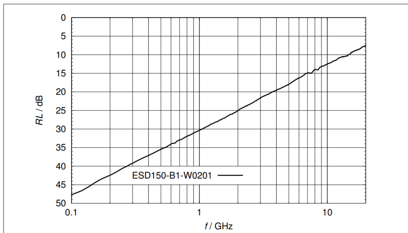
图10 回波损耗 RL = f(f) , 在 50\ \Omega 系统中测量
