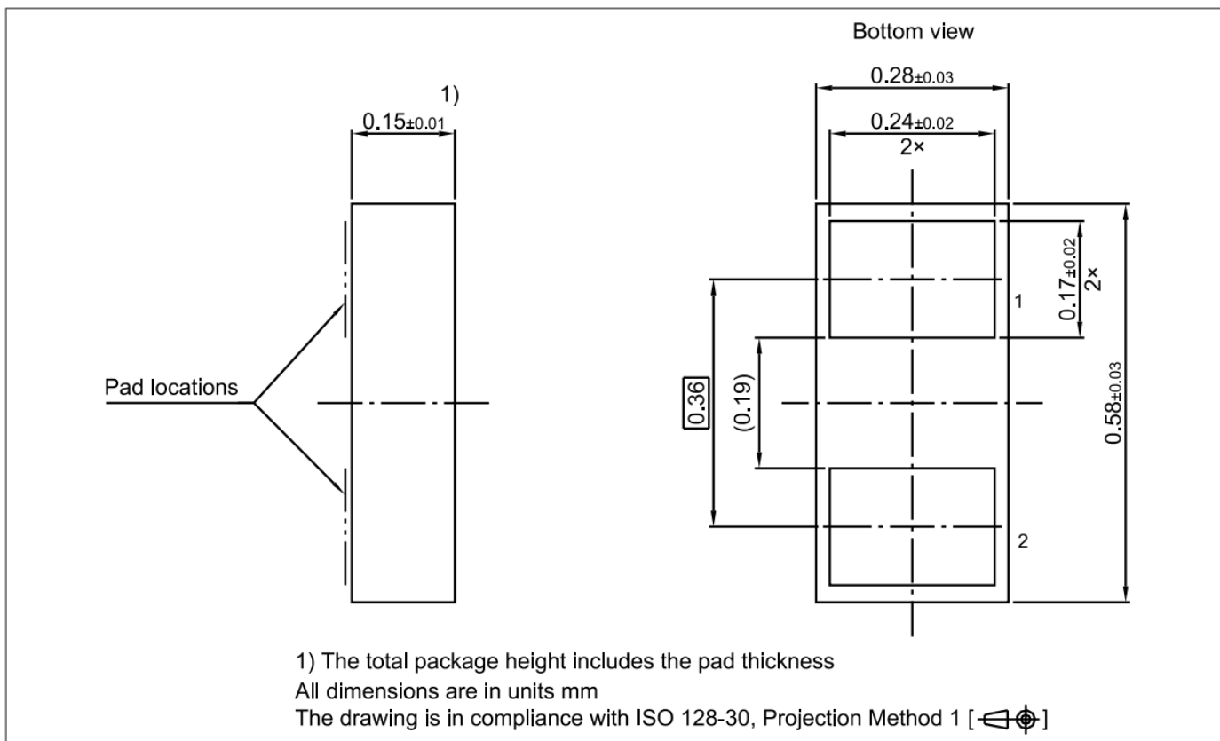
图11 WLL-2-3封装
