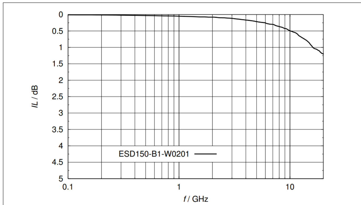
图9 插入损耗: IL = f(f) , 在 50\ \Omega 系统中测量
