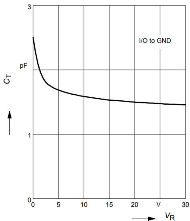
二极管电容 C_T = f(V_R)
