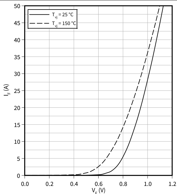
順電圧特性 (typical), 逆極性保護ダイオード B
