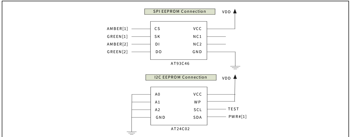
Figure 6 EEPROM 接続の例
