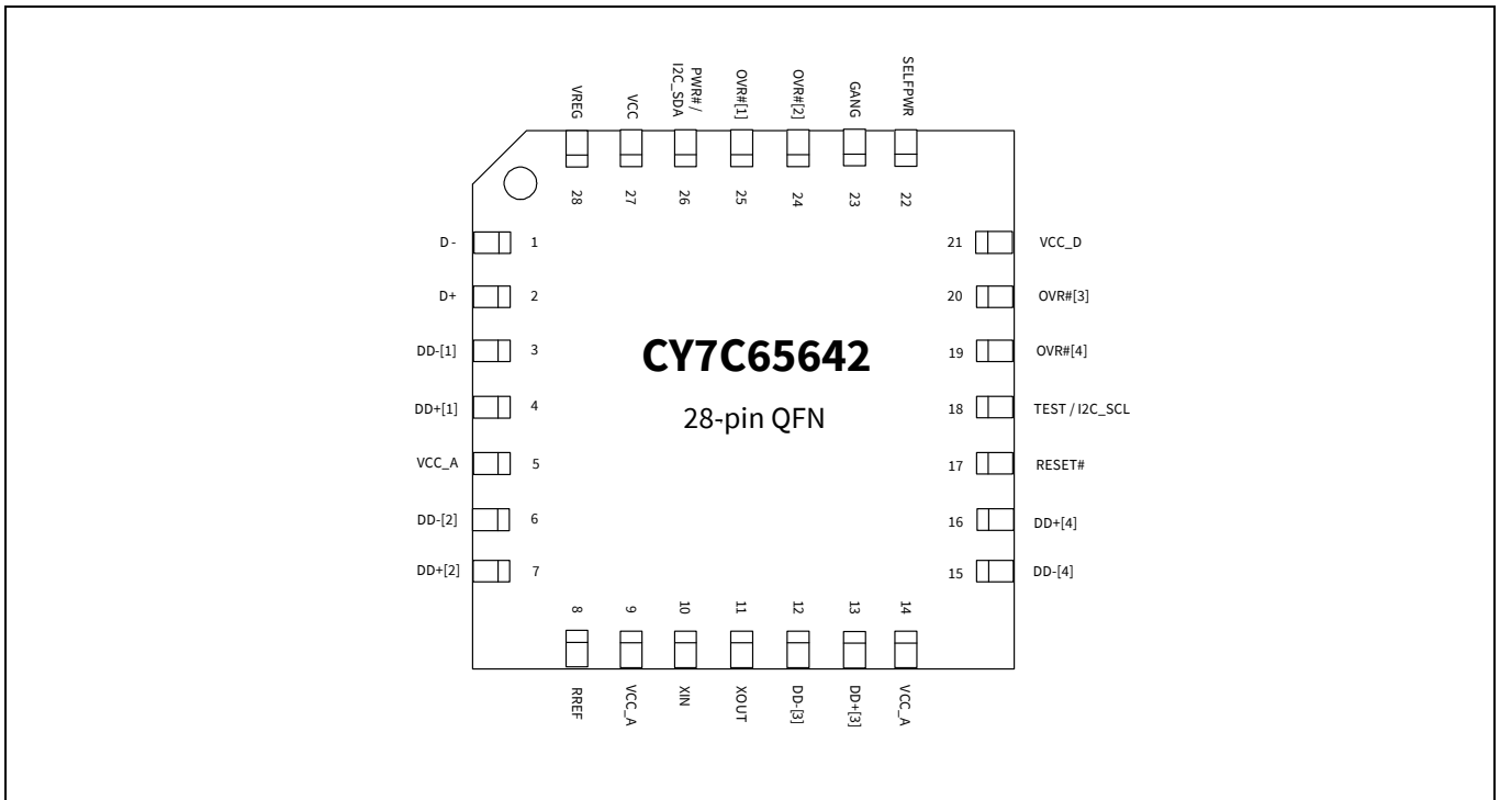
Figure 5 28 ピン QFN (5 × 5 × 0.8 mm) ピン配置
