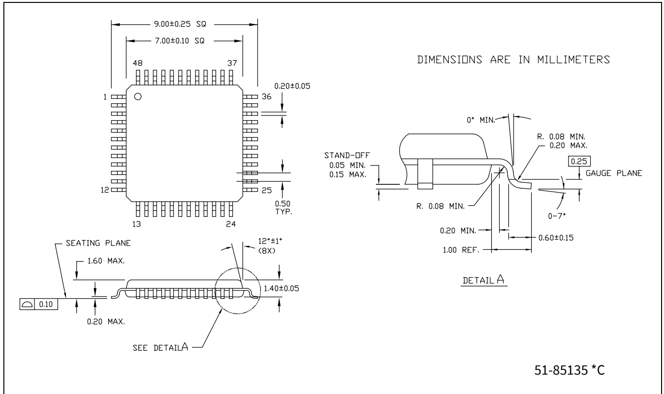
Figure 8 48ピンTQFP (7×7×1.4 mm) A48パッケージ外形図 (PG-TQFP-48)
