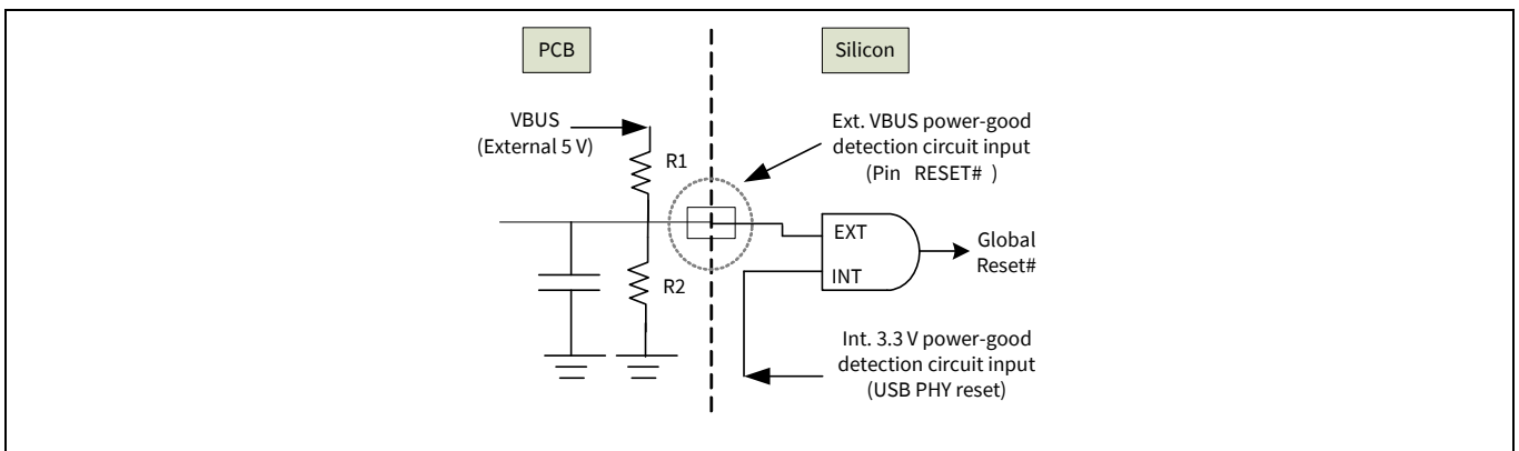
Figure 7 パワーオンリセット
