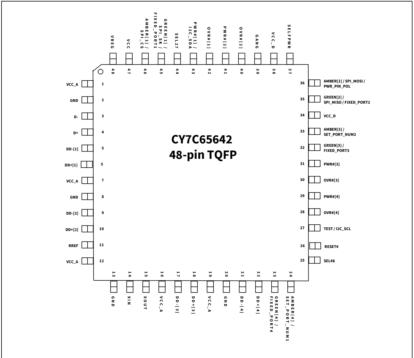
Figure 4 48ピンTQFP (7×7×1.4 mm) ピン配置
