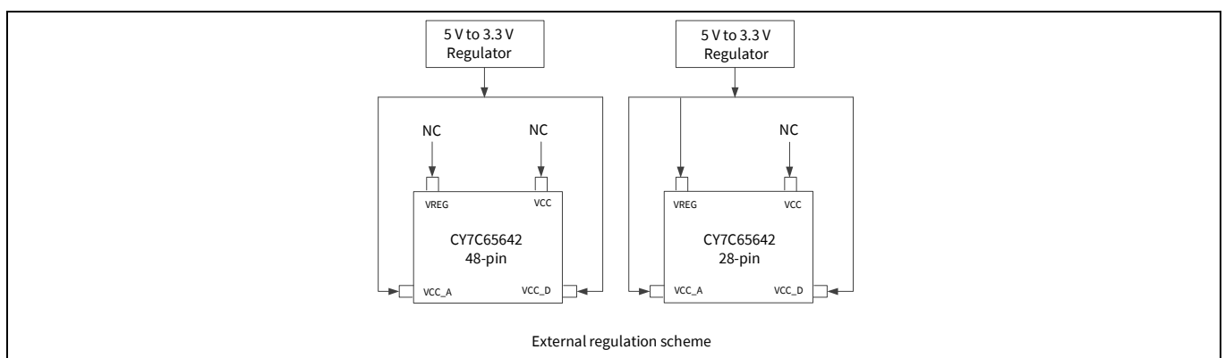
Figure 2 外部レギュレータ使用の場合
