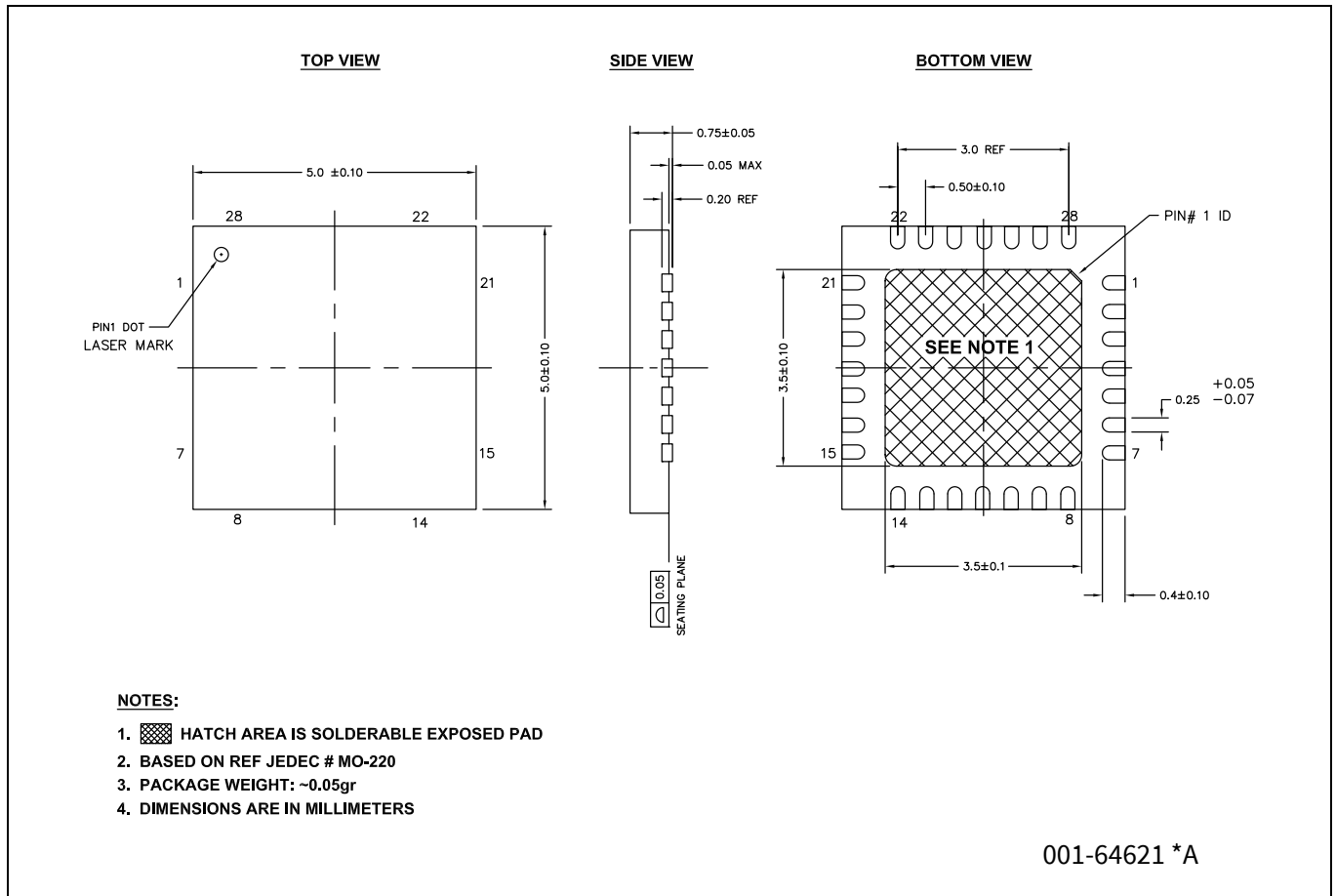
Figure 9 28ピンQFN ((5 × 5 × 0.8 mm) LT28A 3.5 × 3.5 E-Pad (Sawn)) パッケージ外形図 (PG-VQFN-28)
