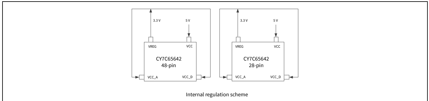
Figure 3 内蔵レギュレータ使用の場合
