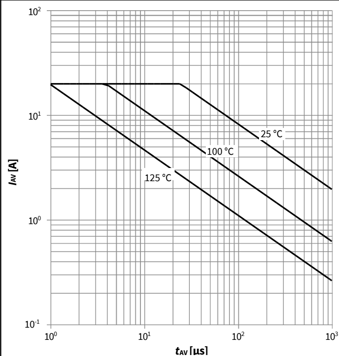
图 13: 雪崩特性
