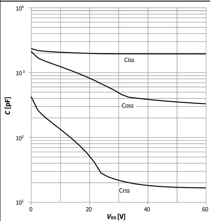
图 11: 典型电容值
