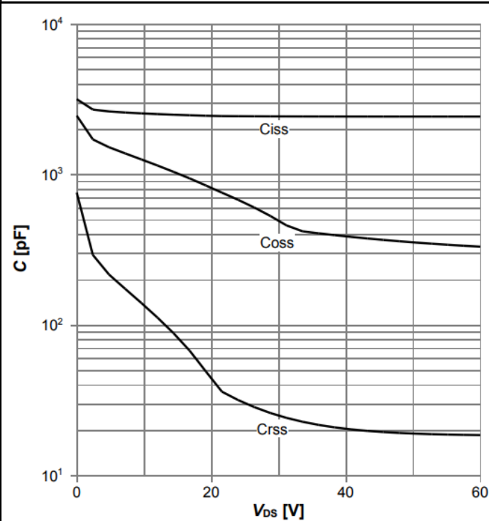
图11：典型电容值
