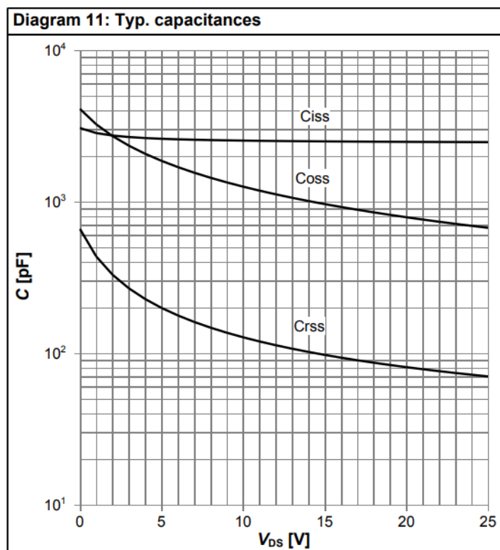
C=f(V_{DS}) ; V_{GS}=0\text{ V} ; f=1\text{ MHz}
