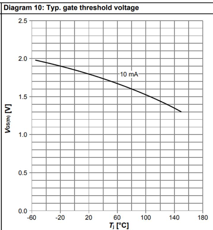
V_{GS(th)}=f(T_j) ; V_{GS}=V_{DS} ; I_D=10\text{ mA}
