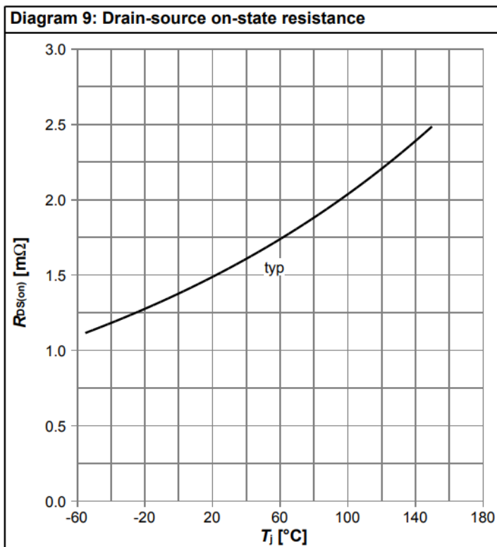
R_{DS(on)}=f(T_j) ; I_D=20\text{ A} ; V_{GS}=10\text{ V}
