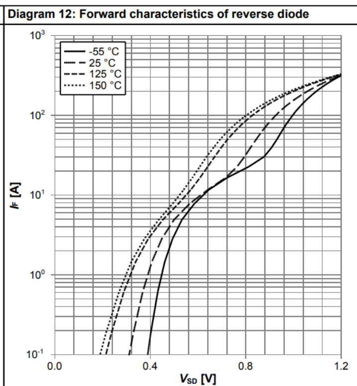
I_F=f(V_{SD}) ; parameter: T_j
