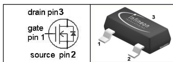
PG-SOT-23
