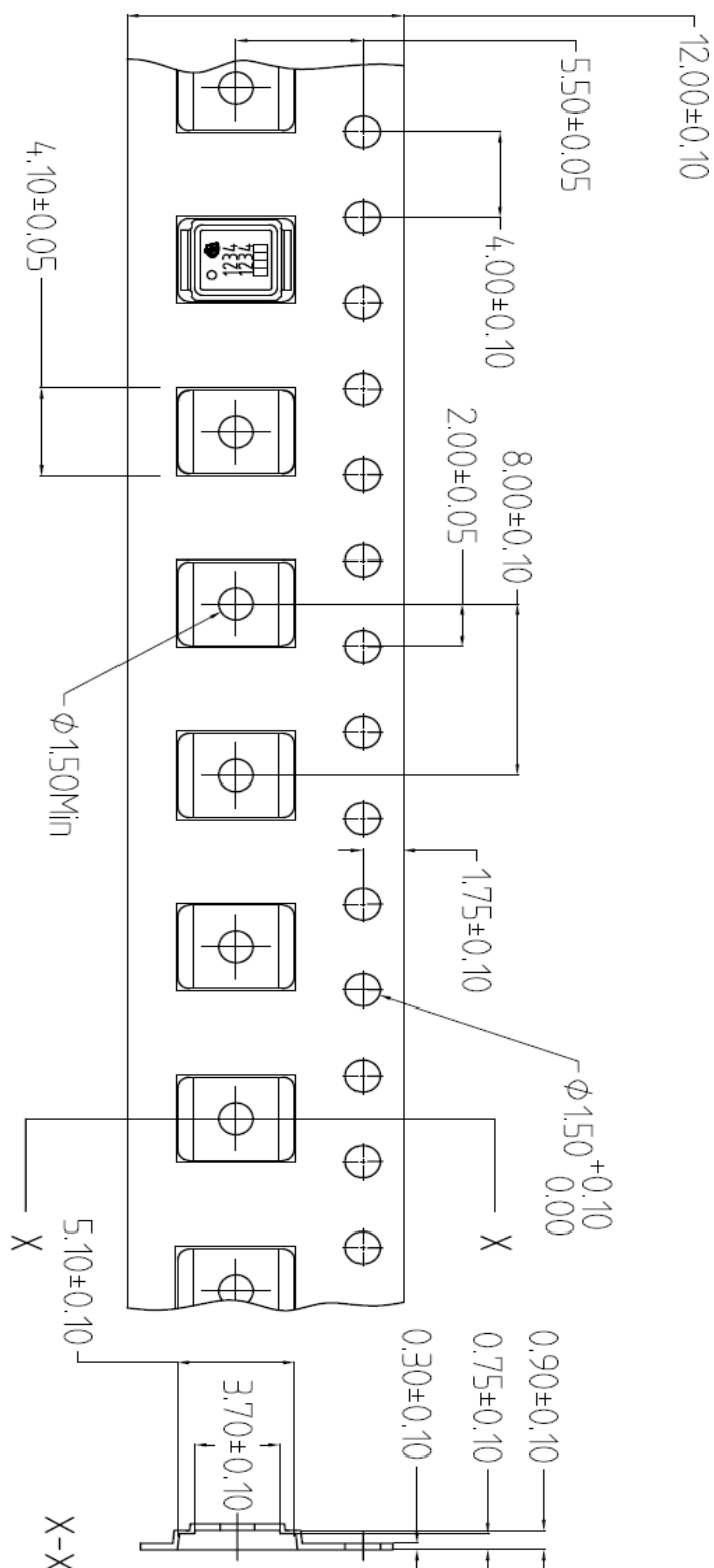
图2 MG-WDSO-2 外形图，尺寸单位为毫米/英寸
