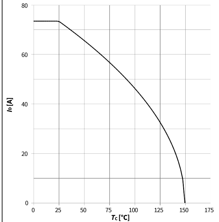
图 2: 漏极电流
