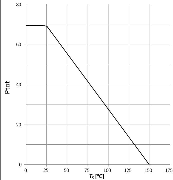
图 1: 功率耗散
