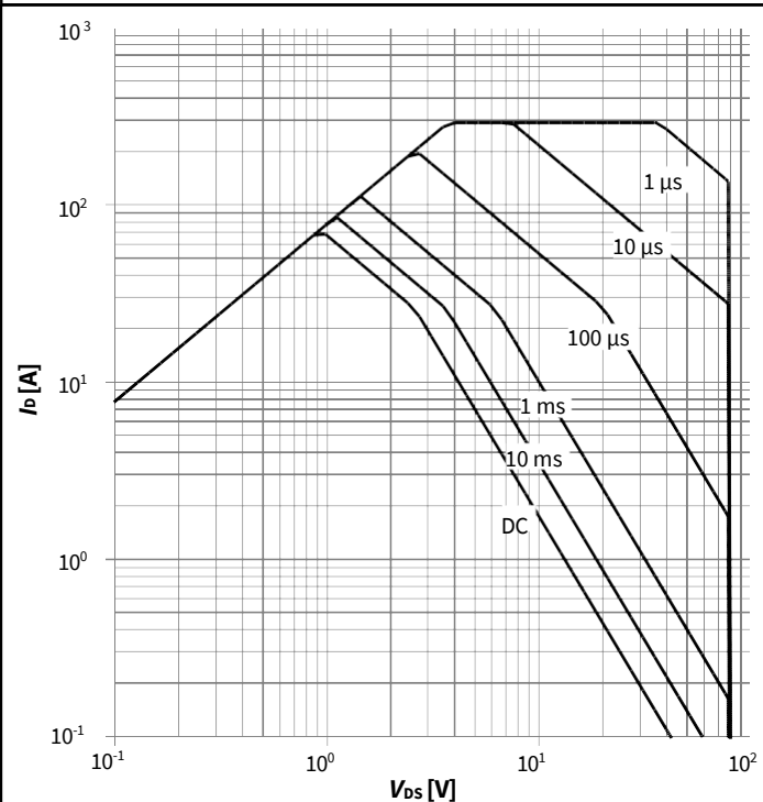
图 3: 安全操作区
