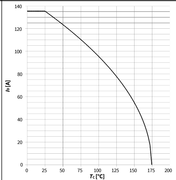
图 2：漏极电流
