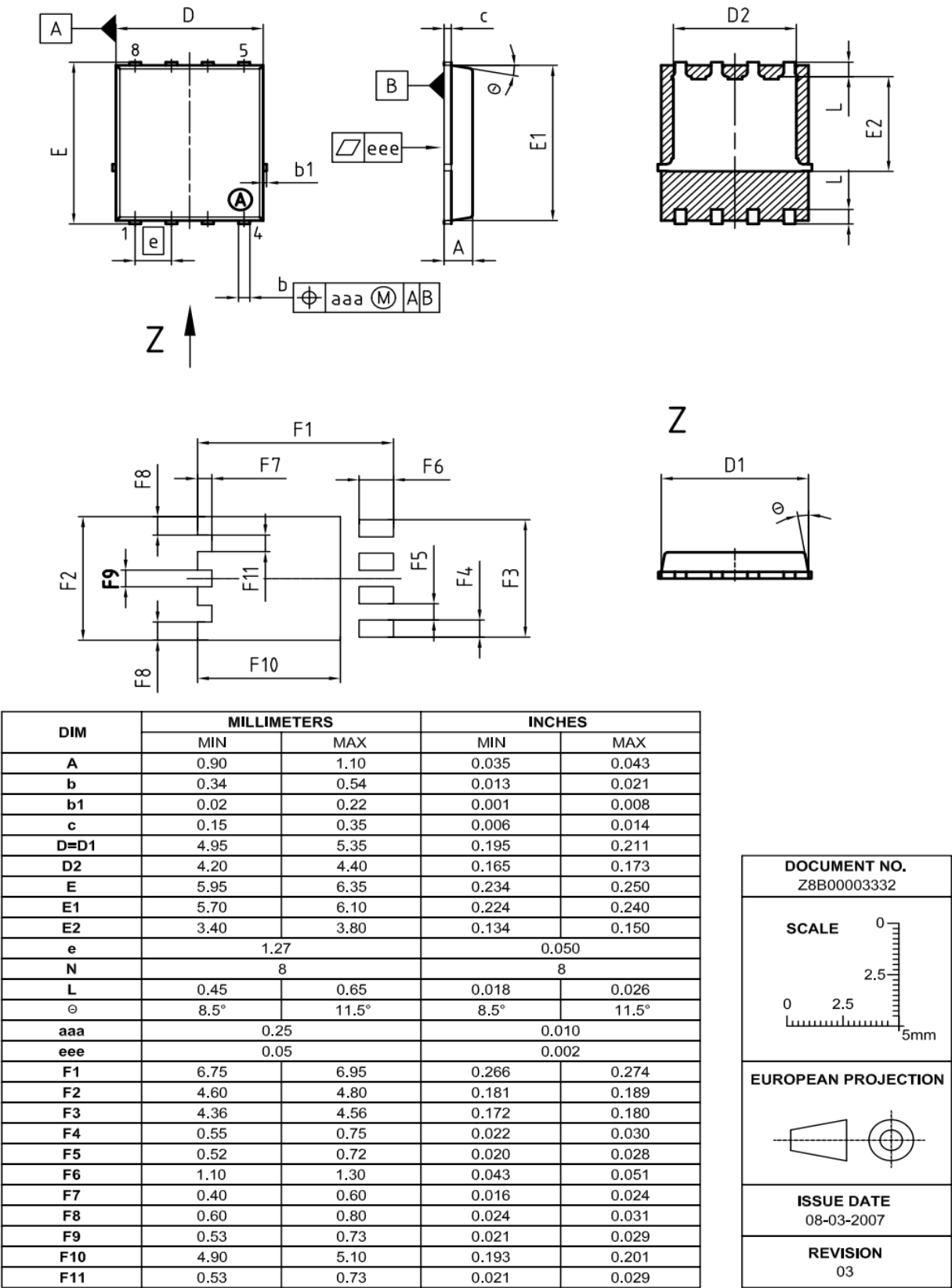
图 1 PG-TDSON-8 外形图, 尺寸单位为毫米
