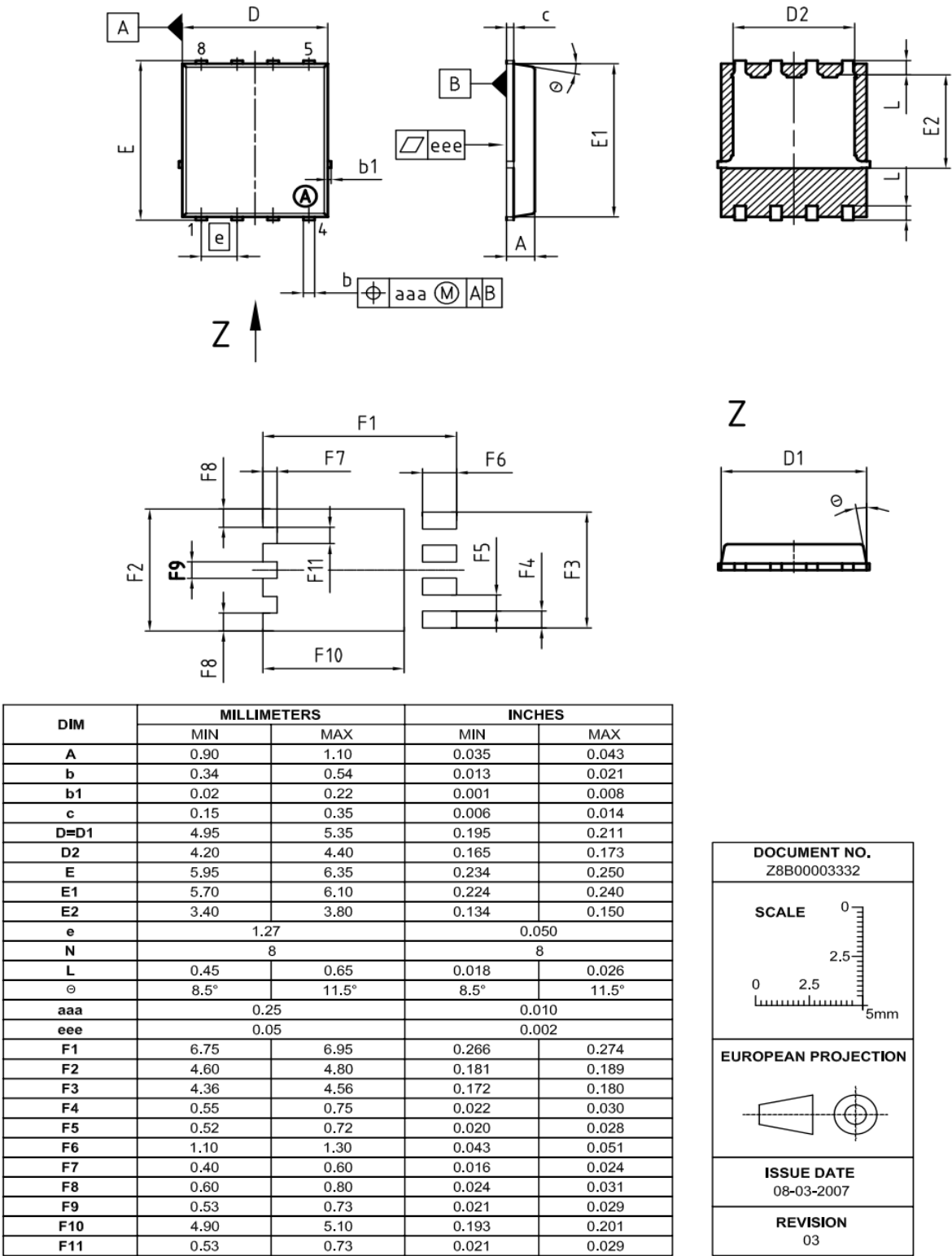
图 1 PG-TDSON-8 外形图，尺寸单位为毫米
