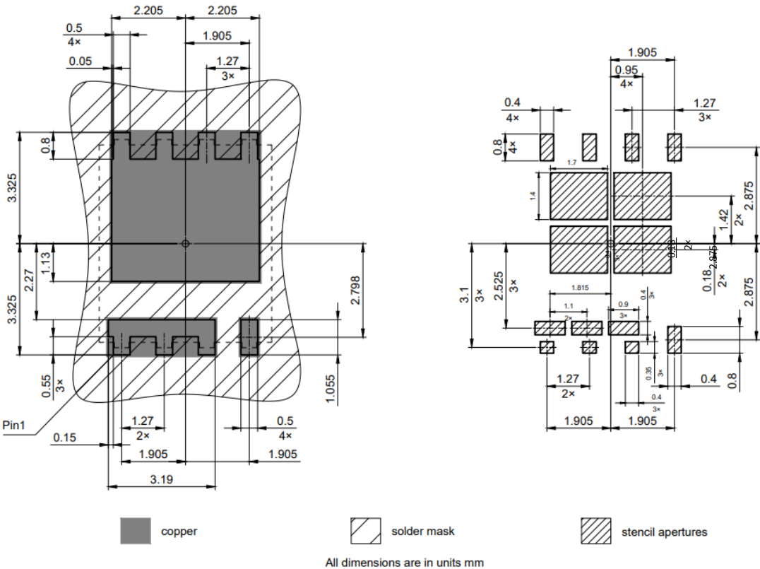
图 2 外形板焊盘 (PG-TDSON-8-FL)，尺寸单位为毫米
