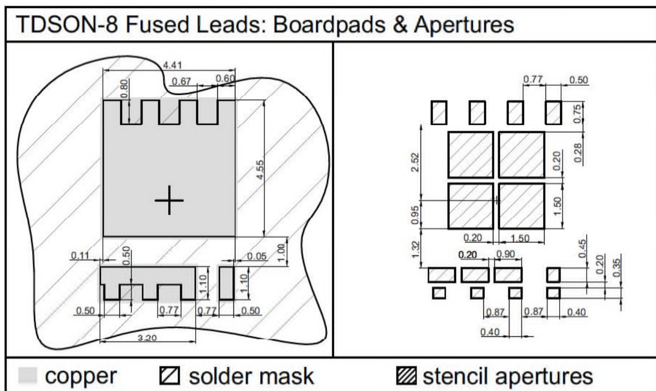
图 2 PG- TDSO N- 8 外形图, 尺寸单位为毫米
