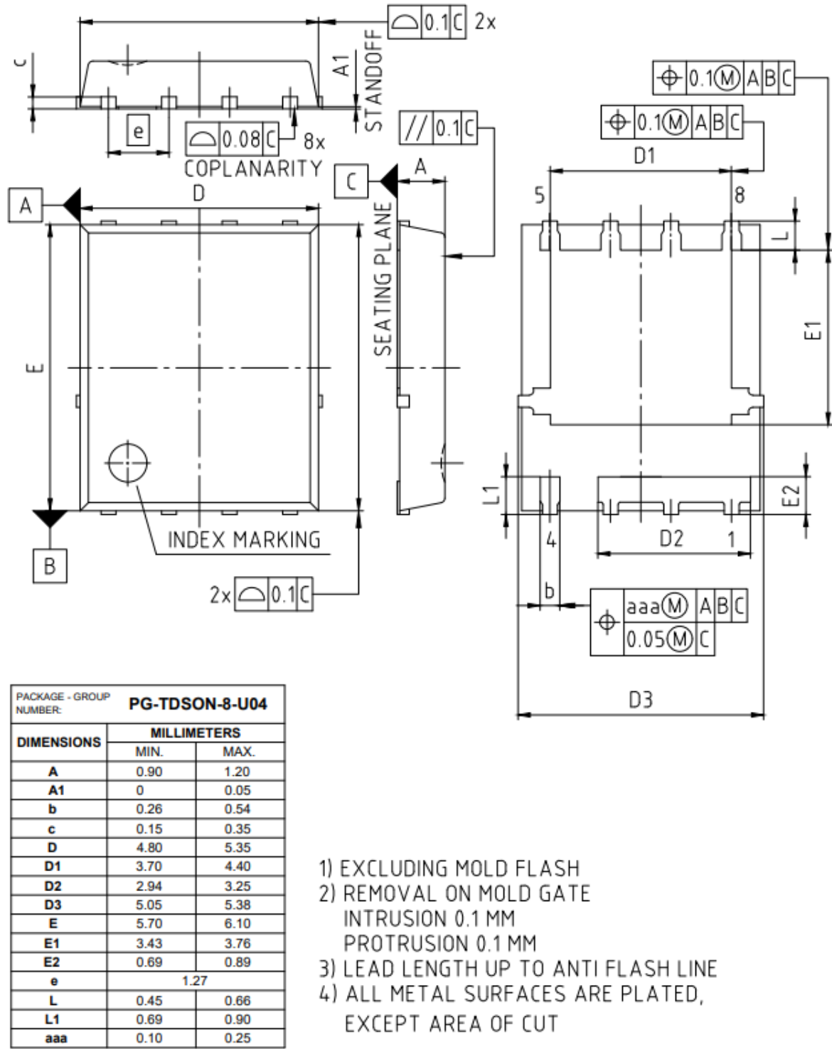
图 1 PG-TDSON-8 FL 外形图，尺寸单位为毫米
