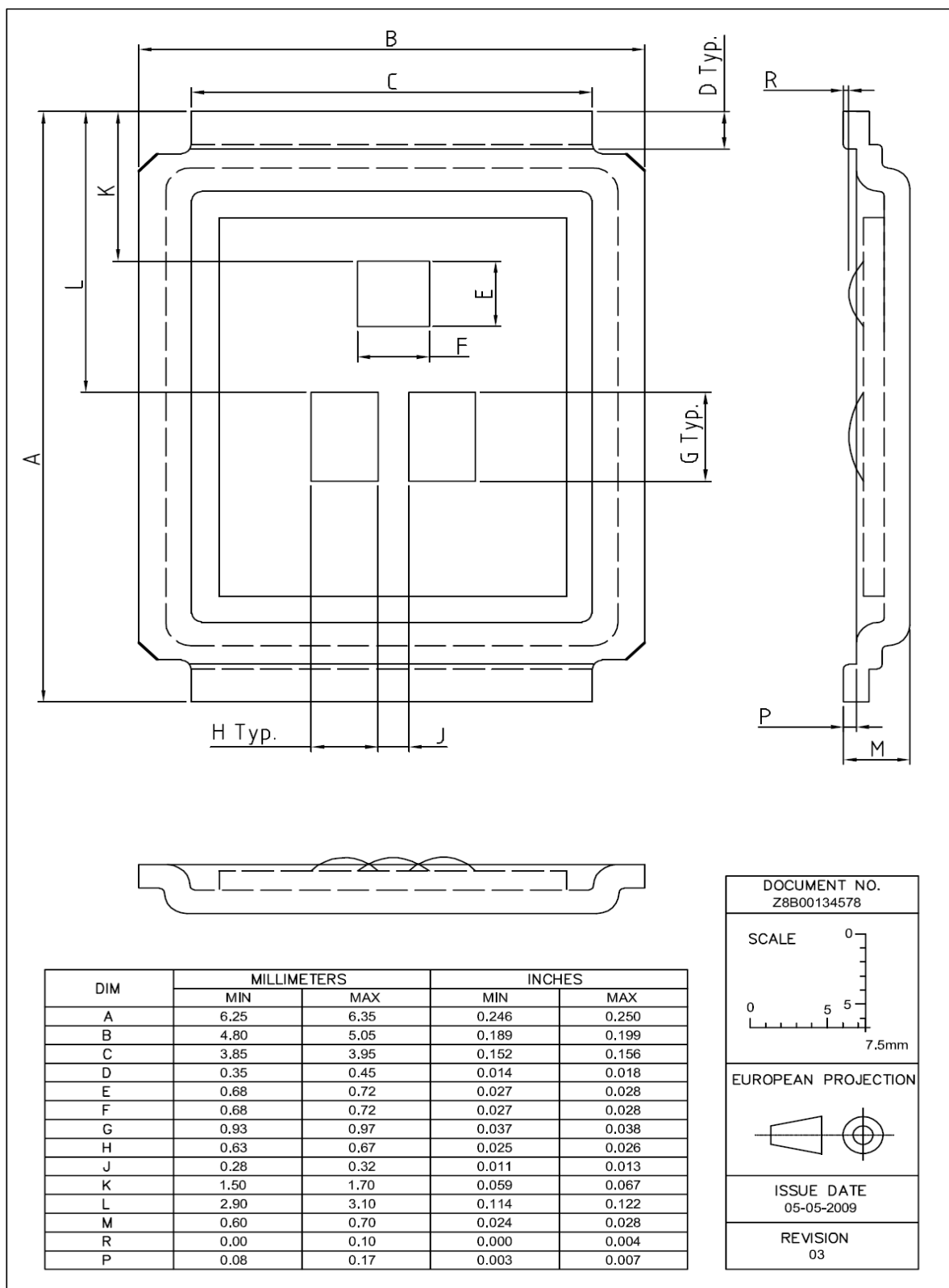
图 1 MG-WDSO-2 外形图，尺寸单位为毫米/英寸
